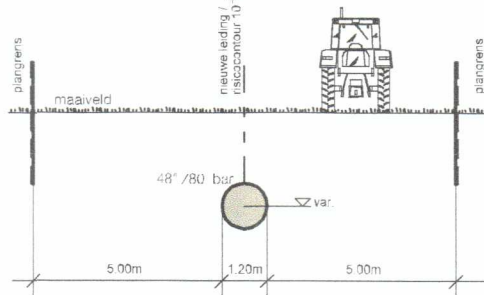
Principe opbouw leidingstrook schaal 1: 200
