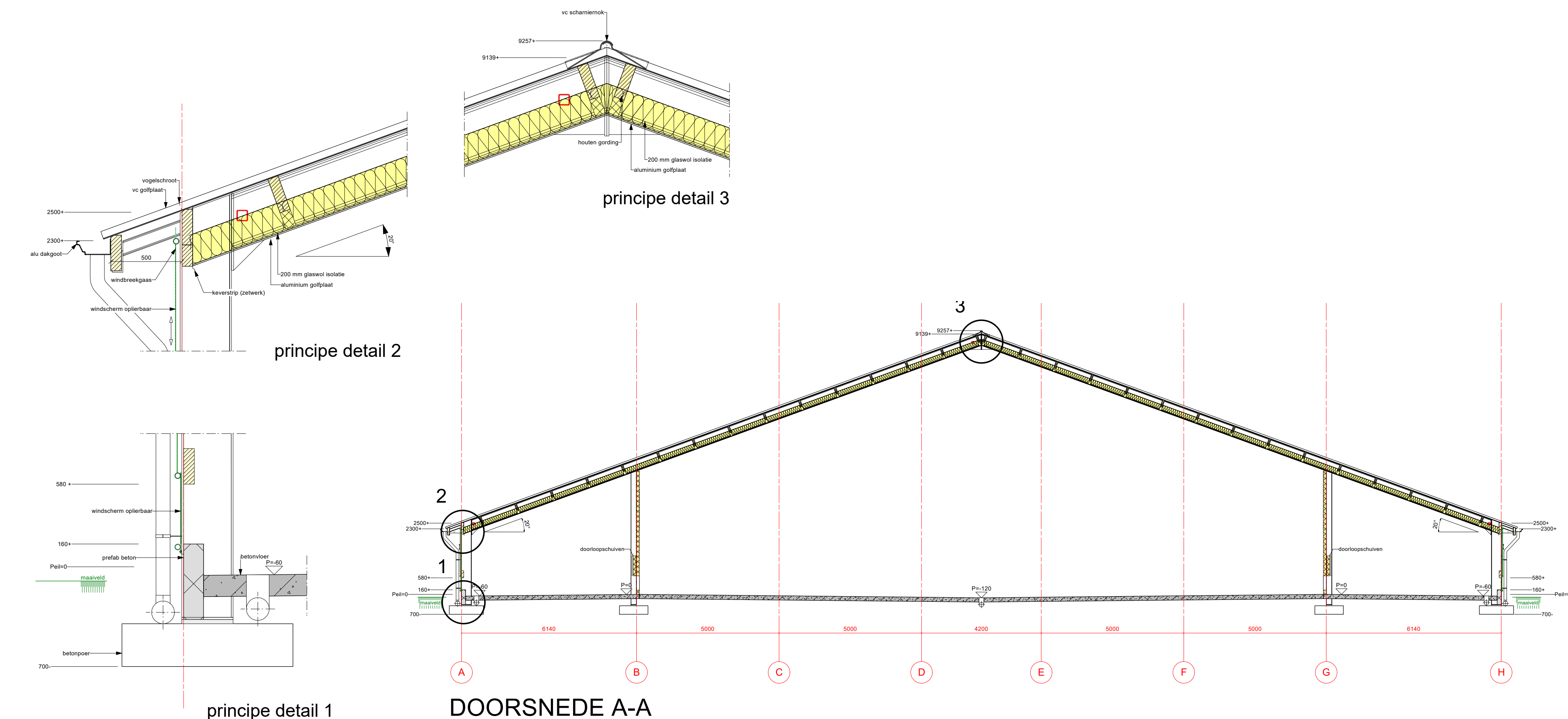
DOORSNEDE A-A
