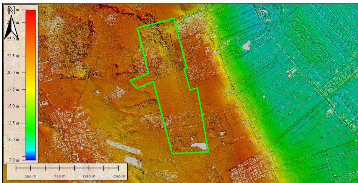
Figuur 10: Overzichtsaafbeelding van de LIDAR in het projectgebied..
