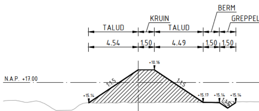
Figuur 2.5: Dwarsprofiel van de wal en houtwal aan de noordoostzijde van het fijnzanddepot
