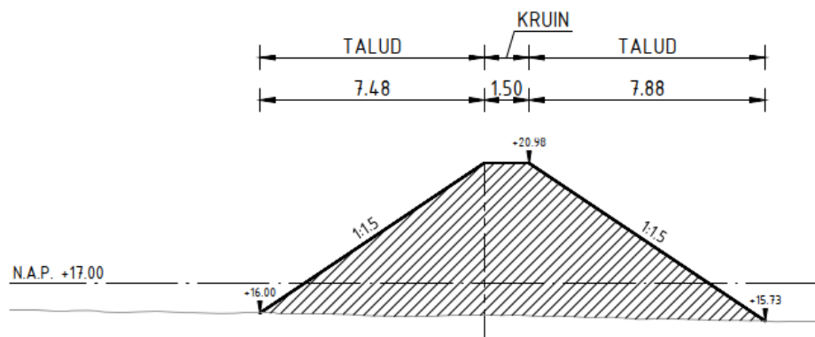
Figuur 2.3: Dwarsprofiel van de wal aan de zijde van de Eeshoornweg en de Veldkampsweg.
