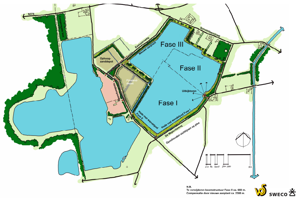
Figuur 1.3: schematische tekening fase III en fijnzanddepot
