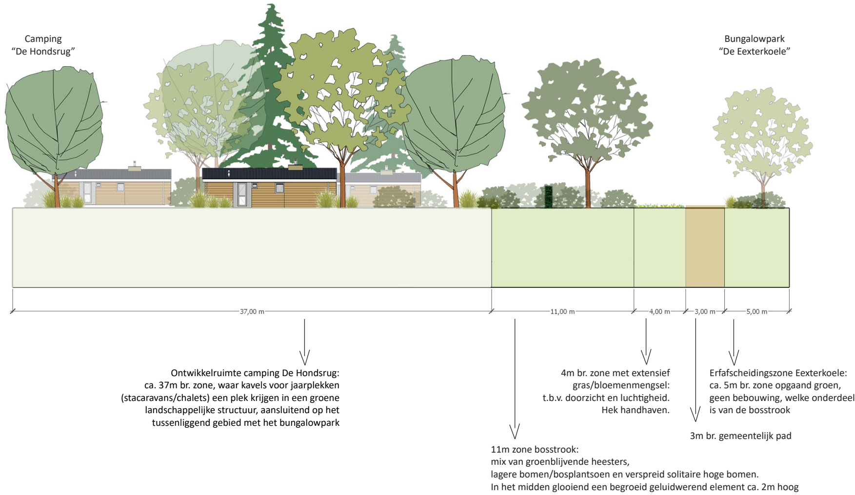
Dwarsprofiel ontwikkelruimte camping (ca. 37m breed) en landschappelijke inpassingszone (ca. 23m breed) tussengebied camping De Hondsrug en bungalowpark De Eexterkoel.
