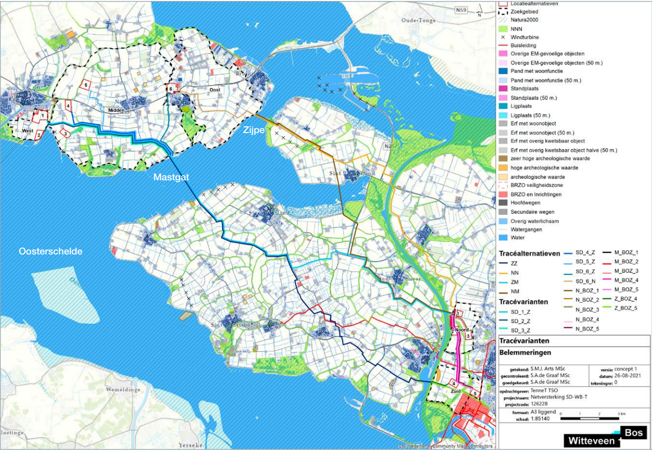
Figuur 2.13 | Overzicht tracéalternatieven en tracévarianten, inclusief belemmeringen.
