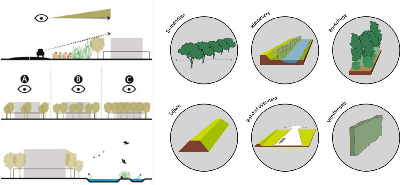
Figuur 4.5 | Oplossingsrichtingen (links) en bouwstenen (rechts) landschappelijke inpassing hoogspanningsstation
