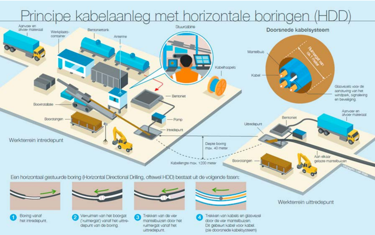
Figuur 5.27 | Situatieschets HDD-boringen (bron: TenneT TSO)
