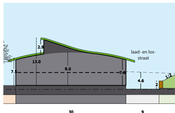
figuur 52 : doorsnede centrumgebouw
