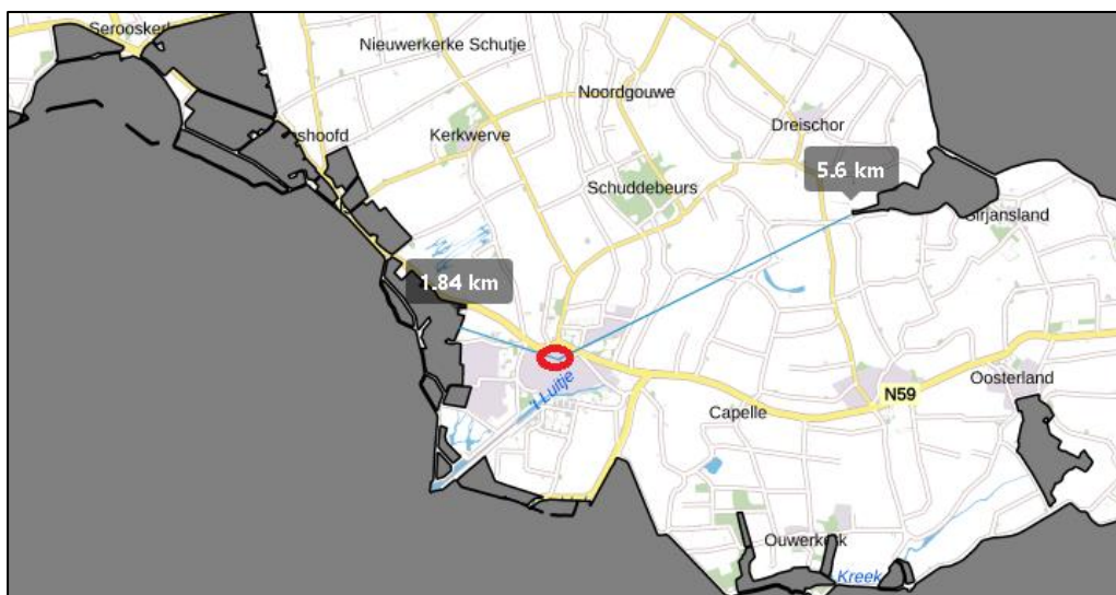
Globale ligging van het plangebied (rood omkaderd) ten opzichte van Natura 2000-gebieden. Bron: PDOK. Bewerking: SAB.
