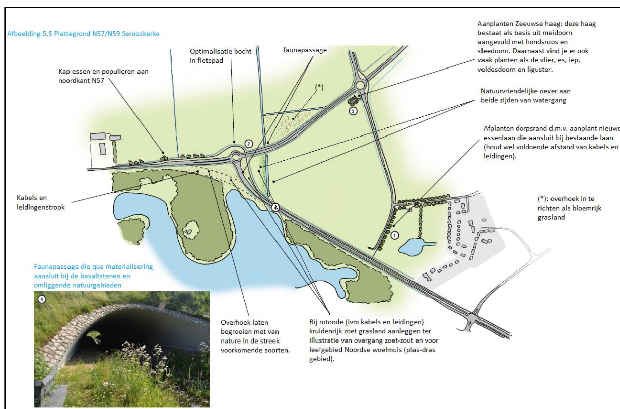
Nieuwe afbeelding 5.5 Plattegrond N57/N59 Serooskerke
