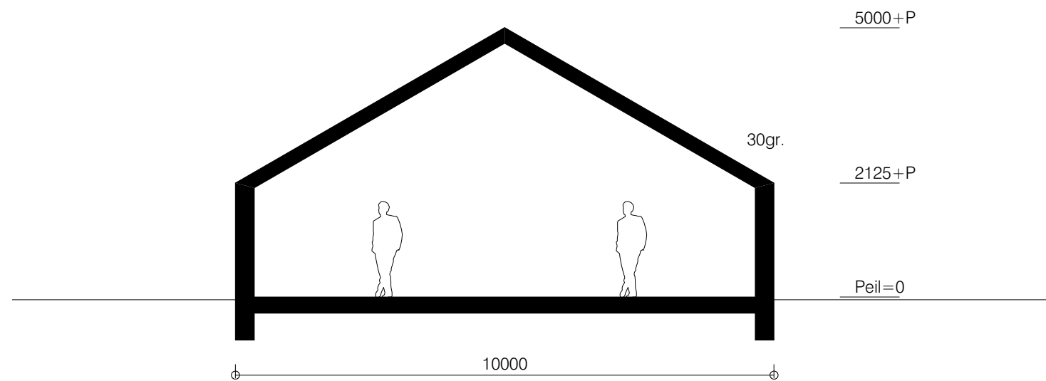
doorsnede
