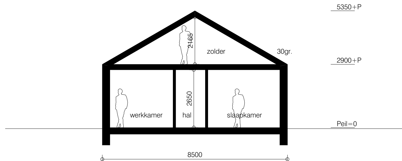
doorsnede
