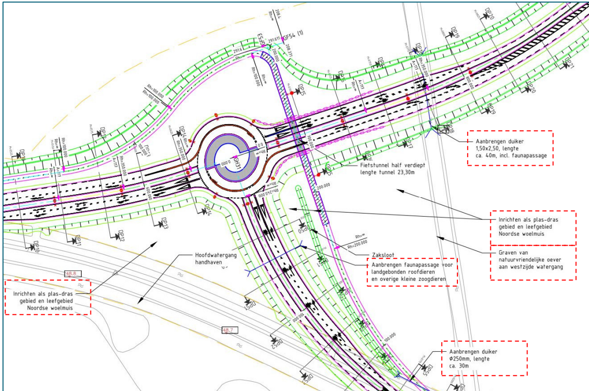
Afbeelding 2.3 Inzoom om ontwerp met flora- en fauna voorzieningen (rood omkaderd)
