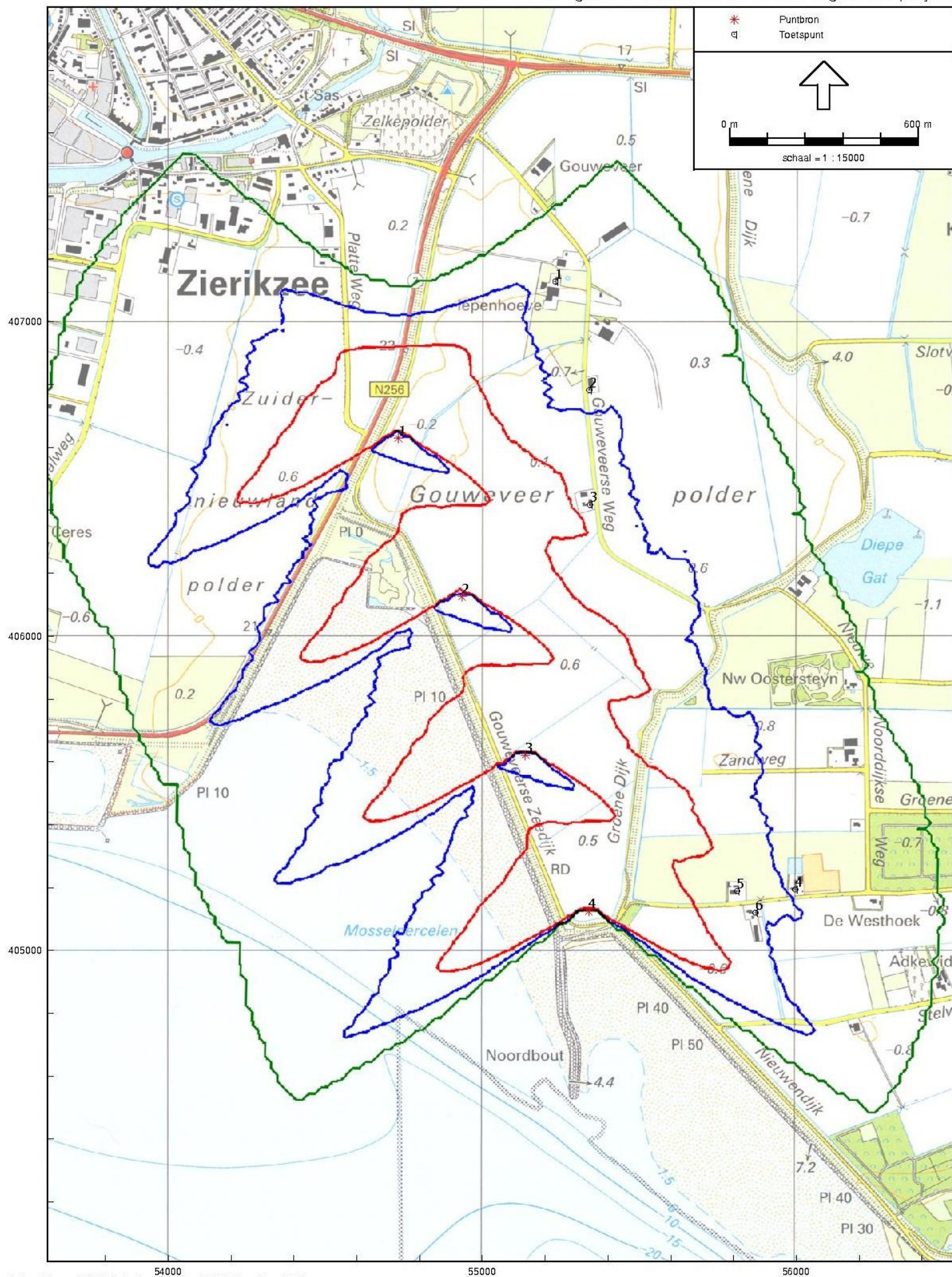
figuur 15 : SWT 2.3-93 schaduwcontouren en rekenpunten
