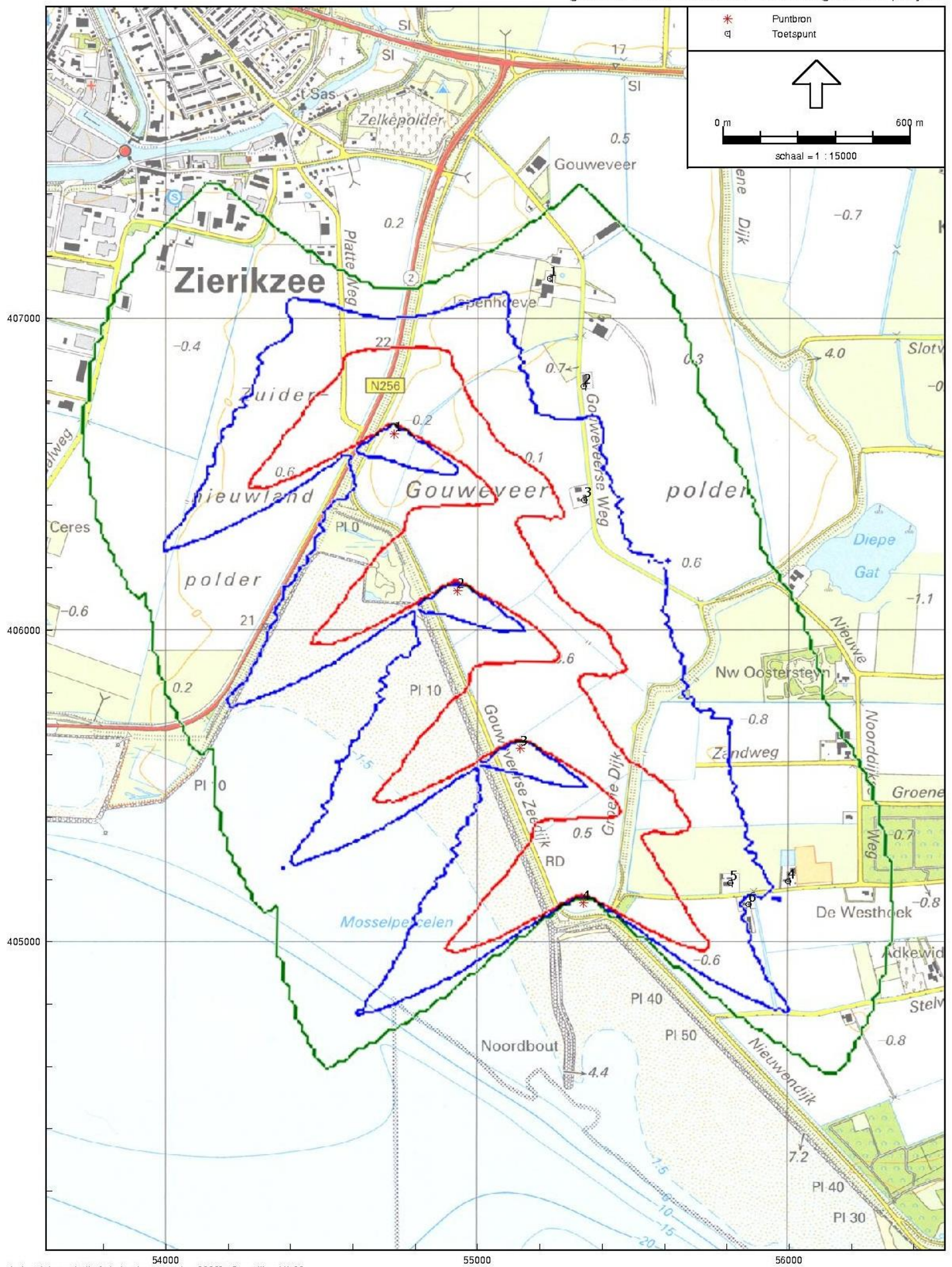
figuur 13 : E-82 schaduwcontouren en rekenpunten
