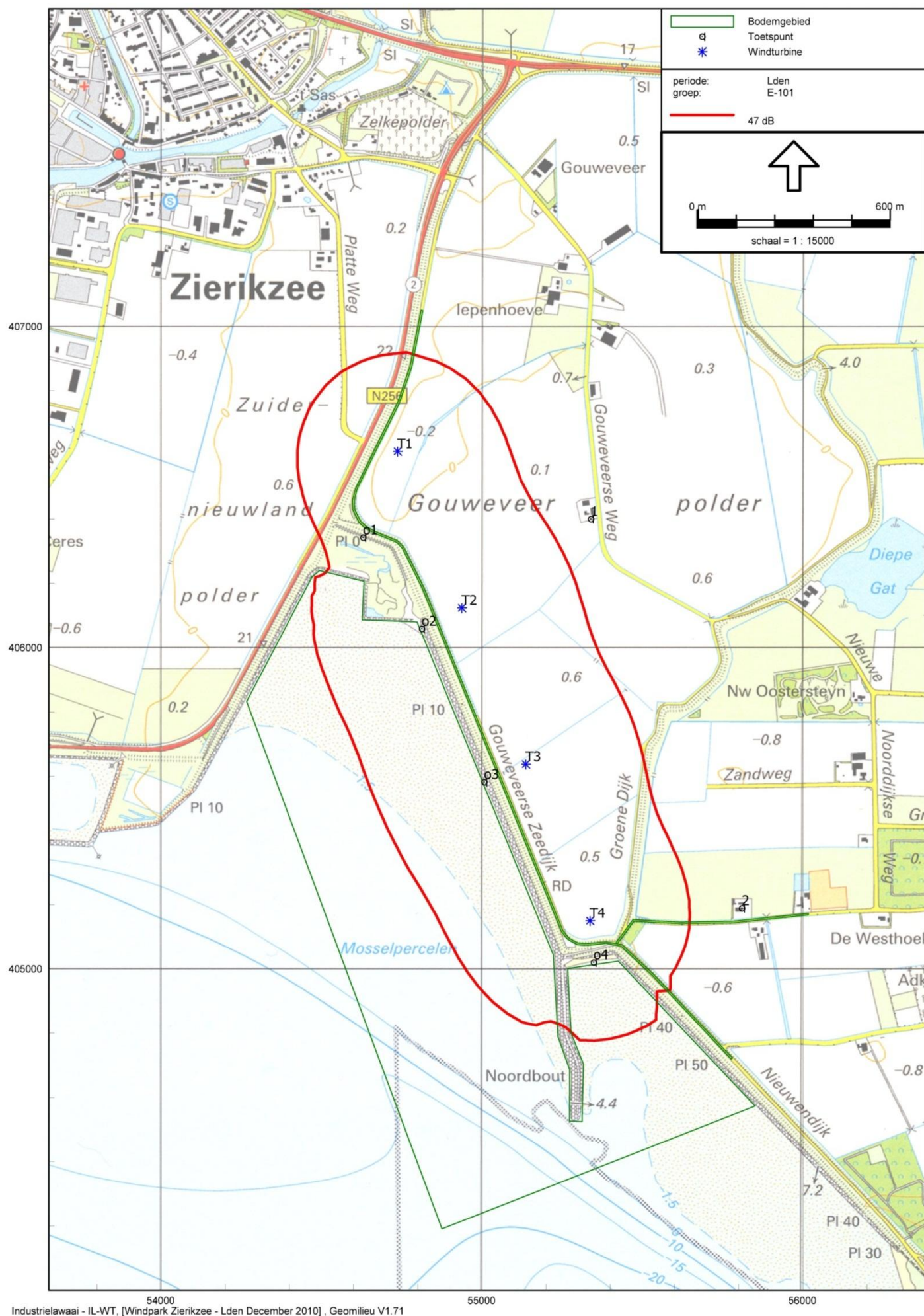
figuur 11 : geluidcontour Enercon E-101 en toetspunten
