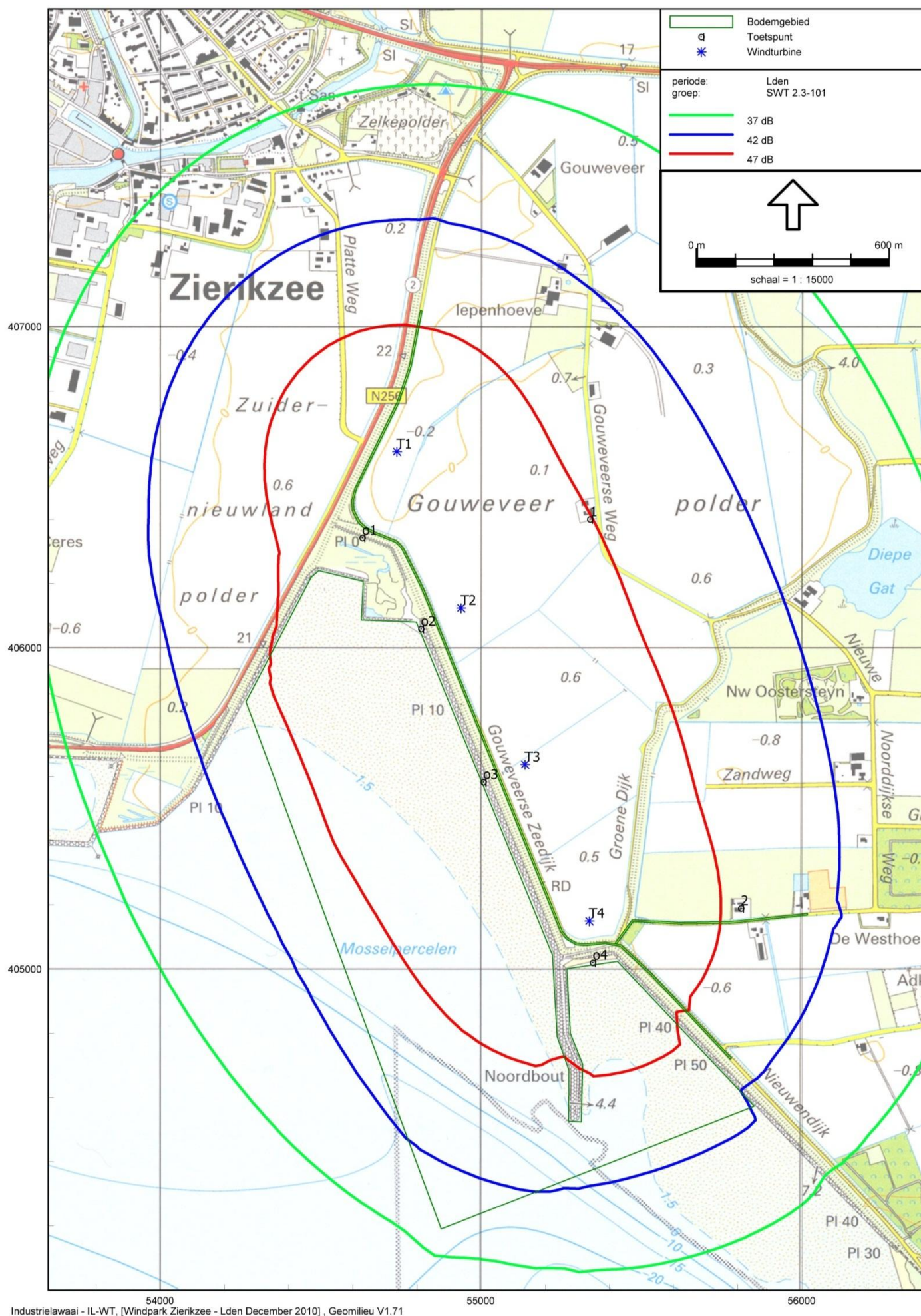
figuur 7 : geluidcontouren SWT 2.3-101 en toetspunten
