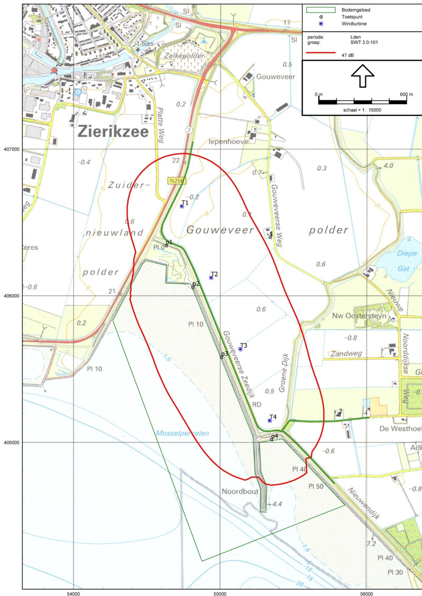
figuur 10 : geluidcontour SWT 3.0-101 en toetspunten
