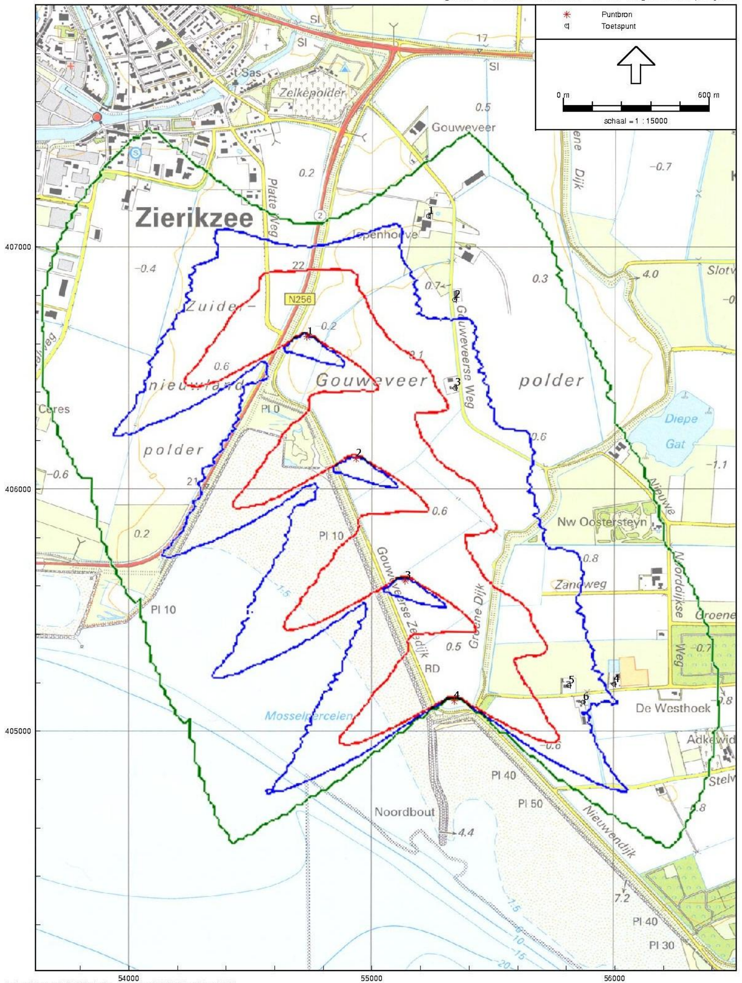
figuur 14 : N90 schaduwcontouren en rekenpunten
