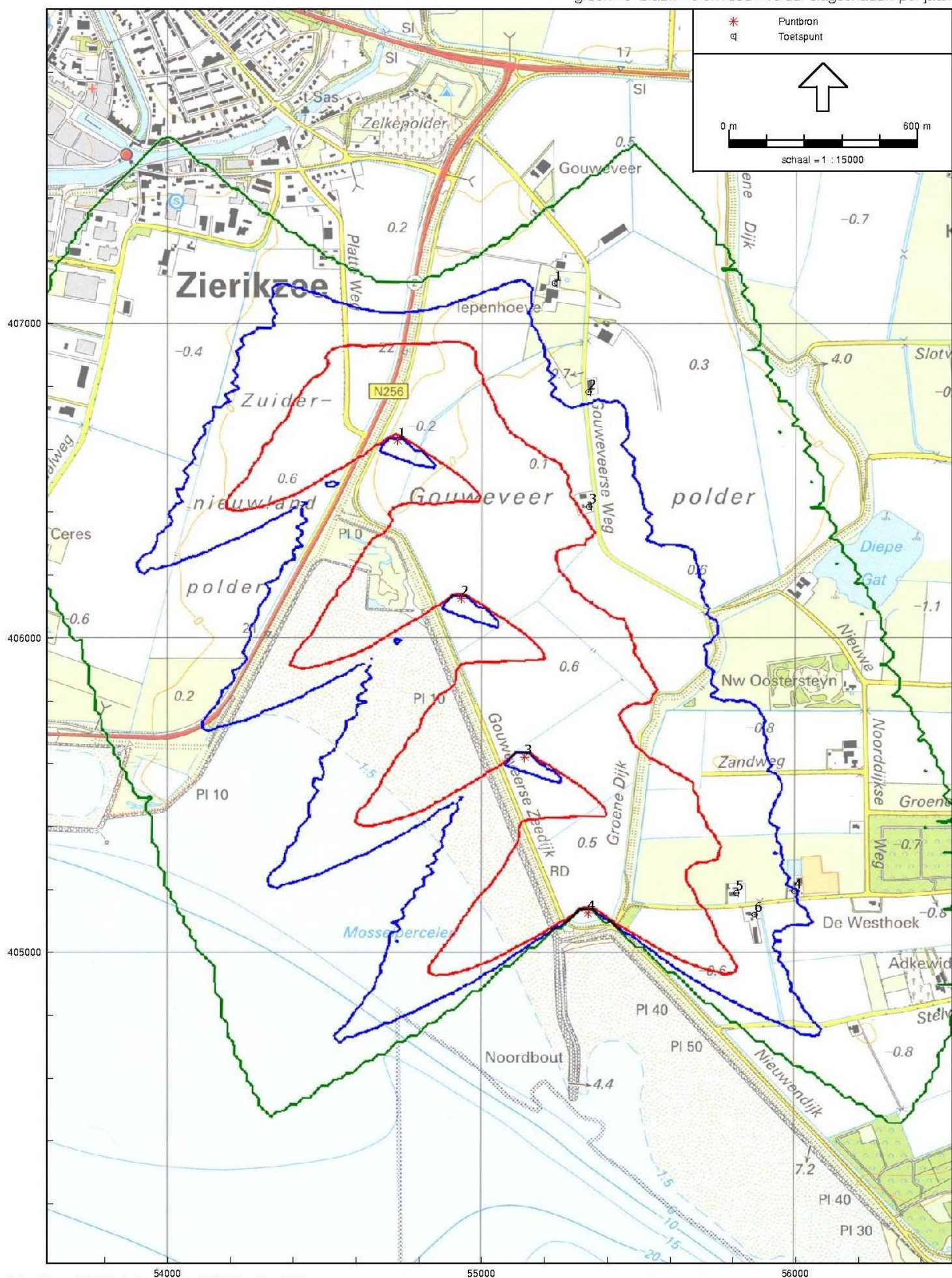
figuur 16 : N100 schaduwcontouren en rekenpunten
