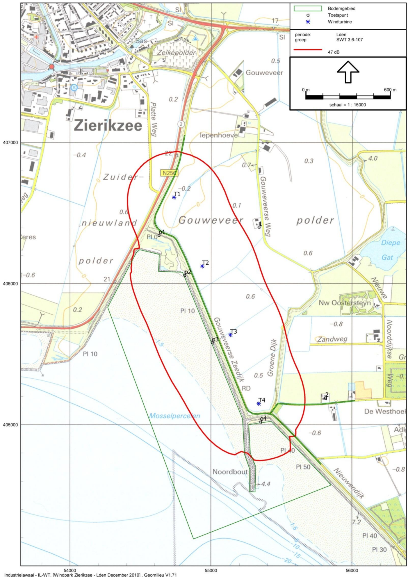
figuur 12 : geluidcontour SWT 3.6-107 en toetspunten
