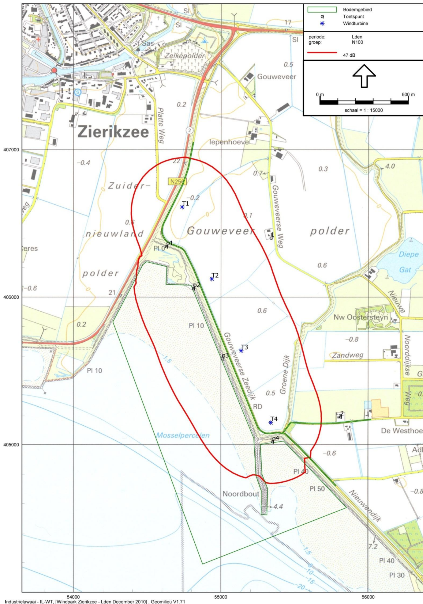
figuur 6 : geluidcontour N100/2500 en toetspunten
