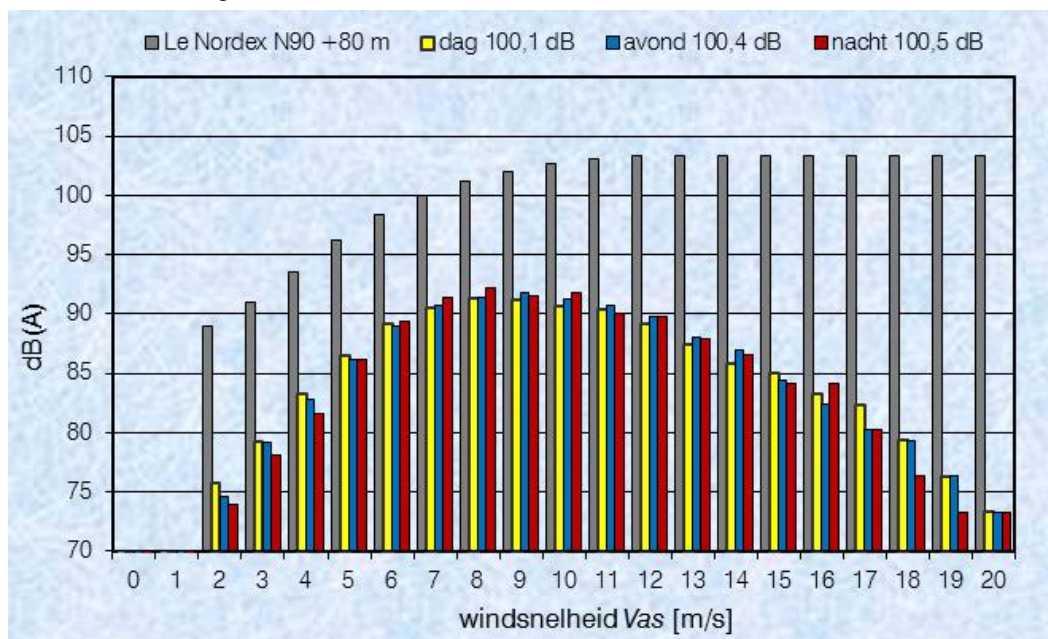
Grafiek 2-4: verdeling bronsterkten Nordex N90/2500
