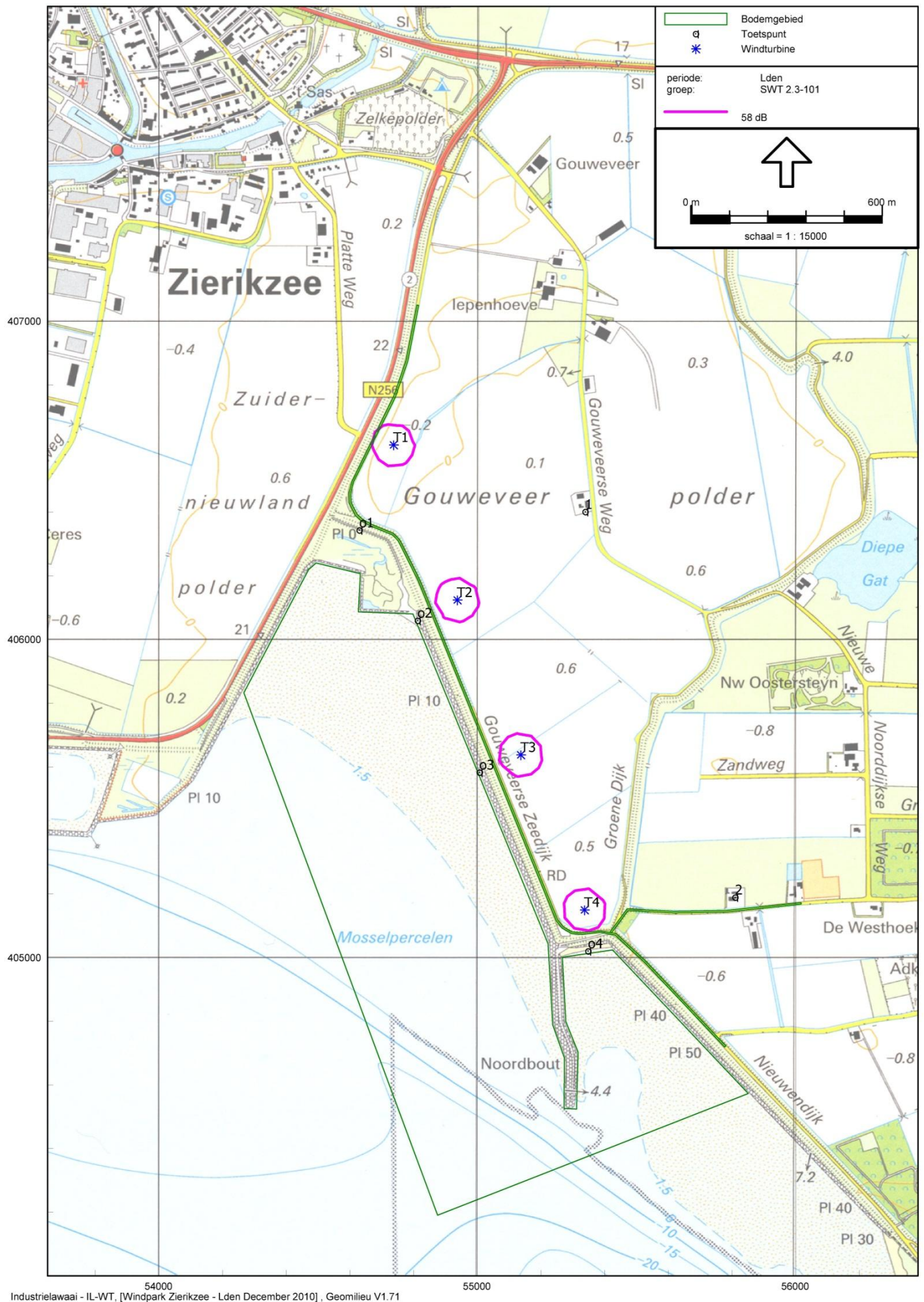
figuur 9 : geluidcontour +1,5 m SWT 2.3-101 en toetspunten
