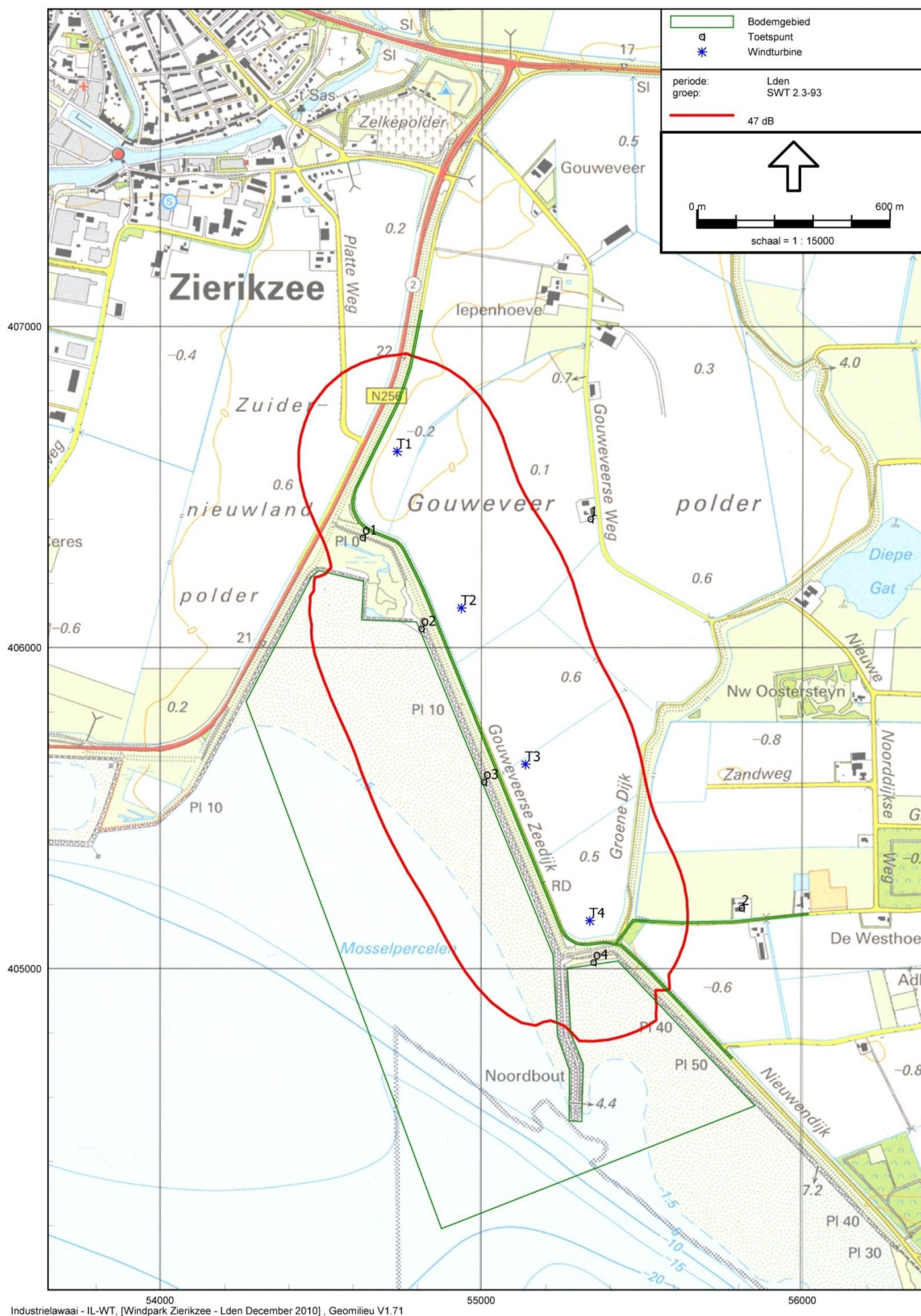
figuur 5 : geluidcontour SWT 2.3-93 en toetspunten
