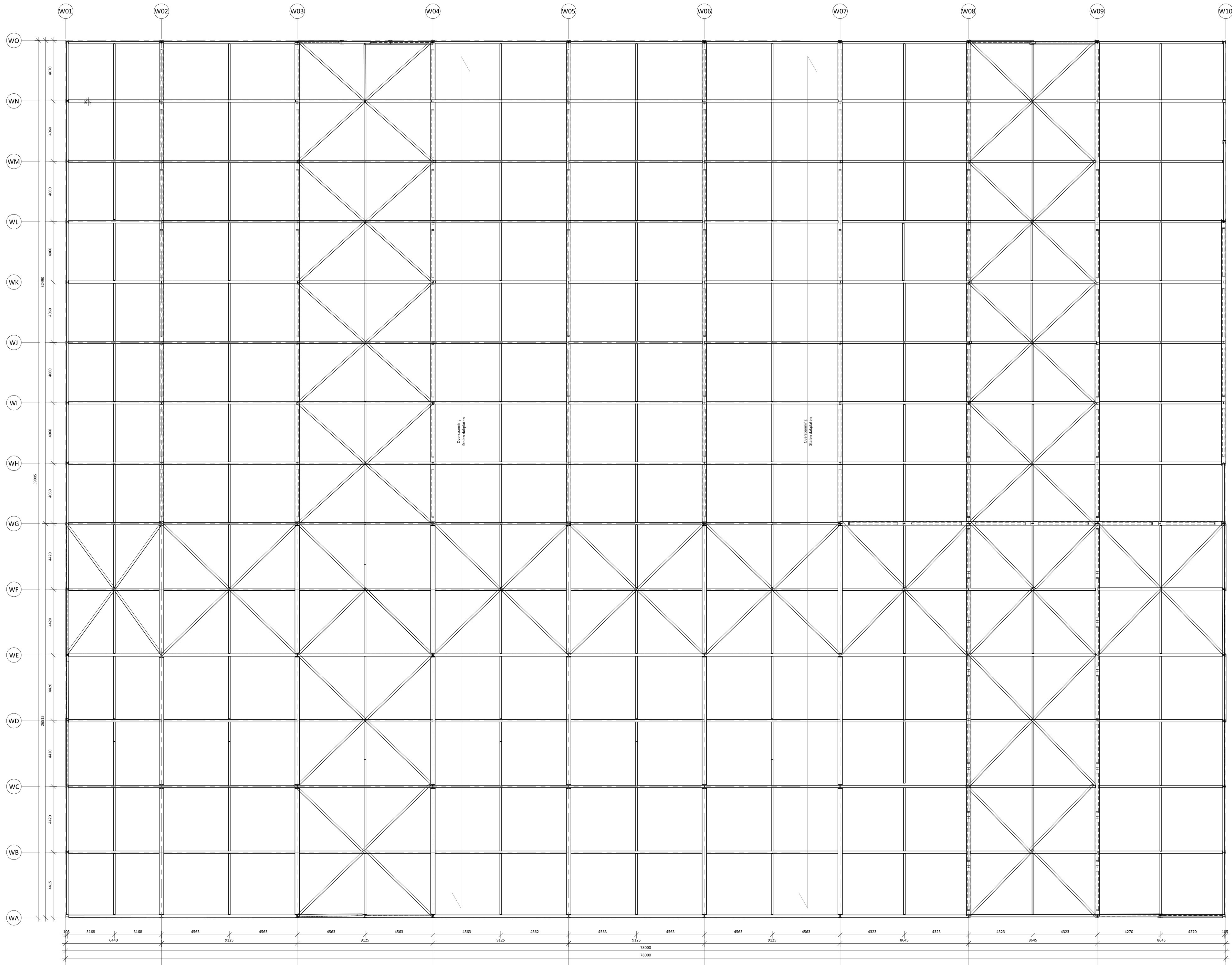
Staalconstructie dak Schaal: 1 : 100
