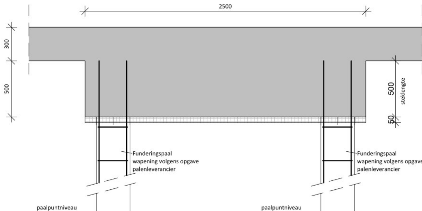
Principe detail twee-/vier paalspoer Schaal: 1 : 20
