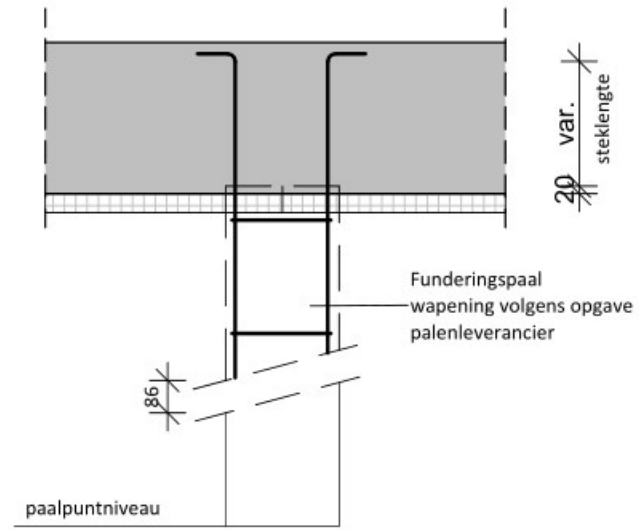
Principe detail paal-vloer Schaal: 1 : 20
