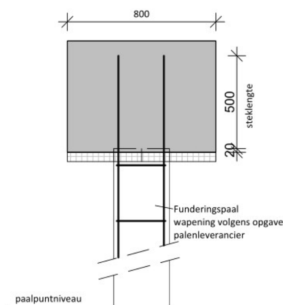
Principe detail paalspoer Schaal: 1 : 20
