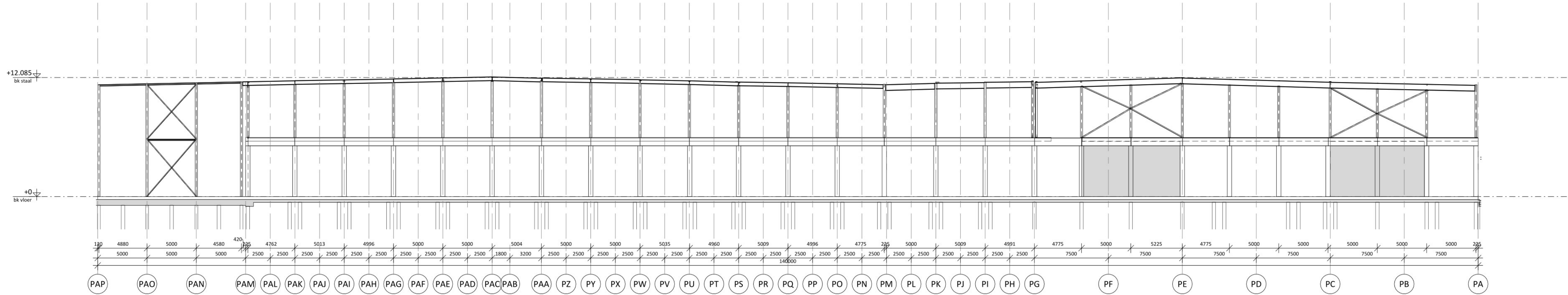
Aanzicht constructie stramien P01
