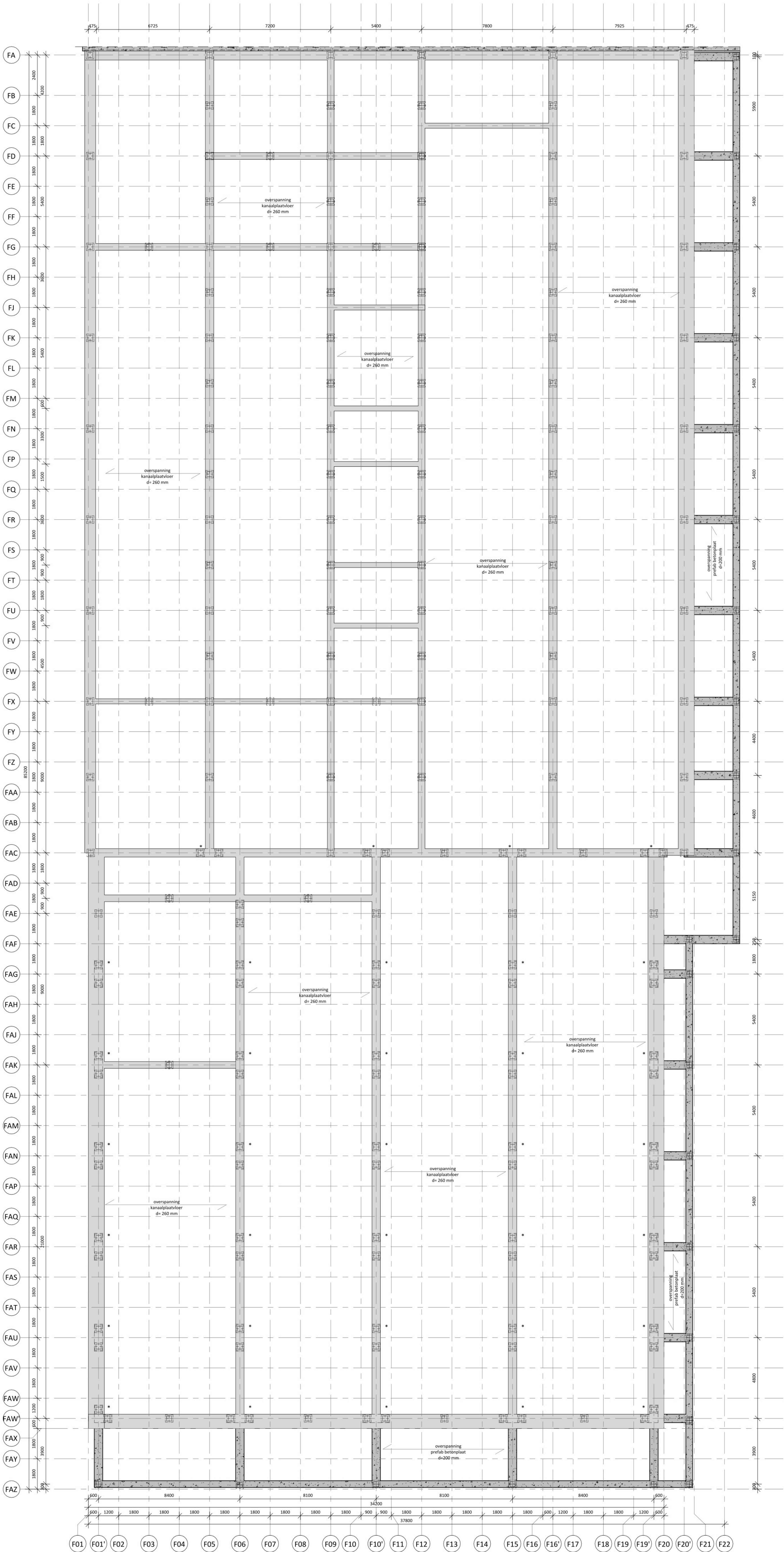
Fundering en palenplan Schaal: 1 : 100 * = twee-paals poer
