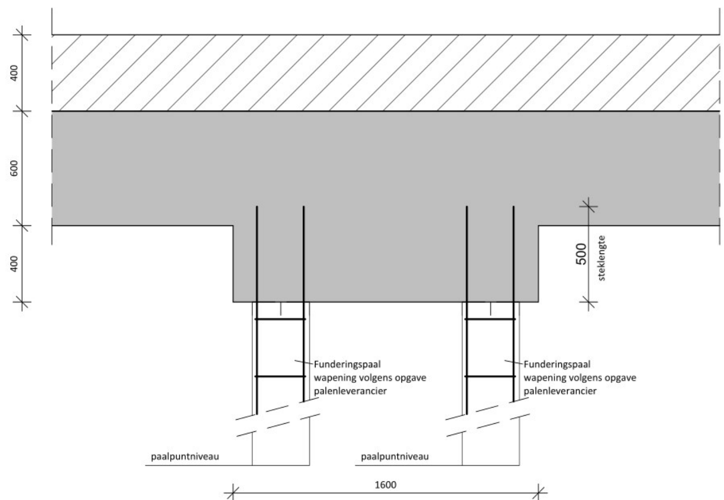
Principe detail tweepaalspoer Schaal: 1 : 20
