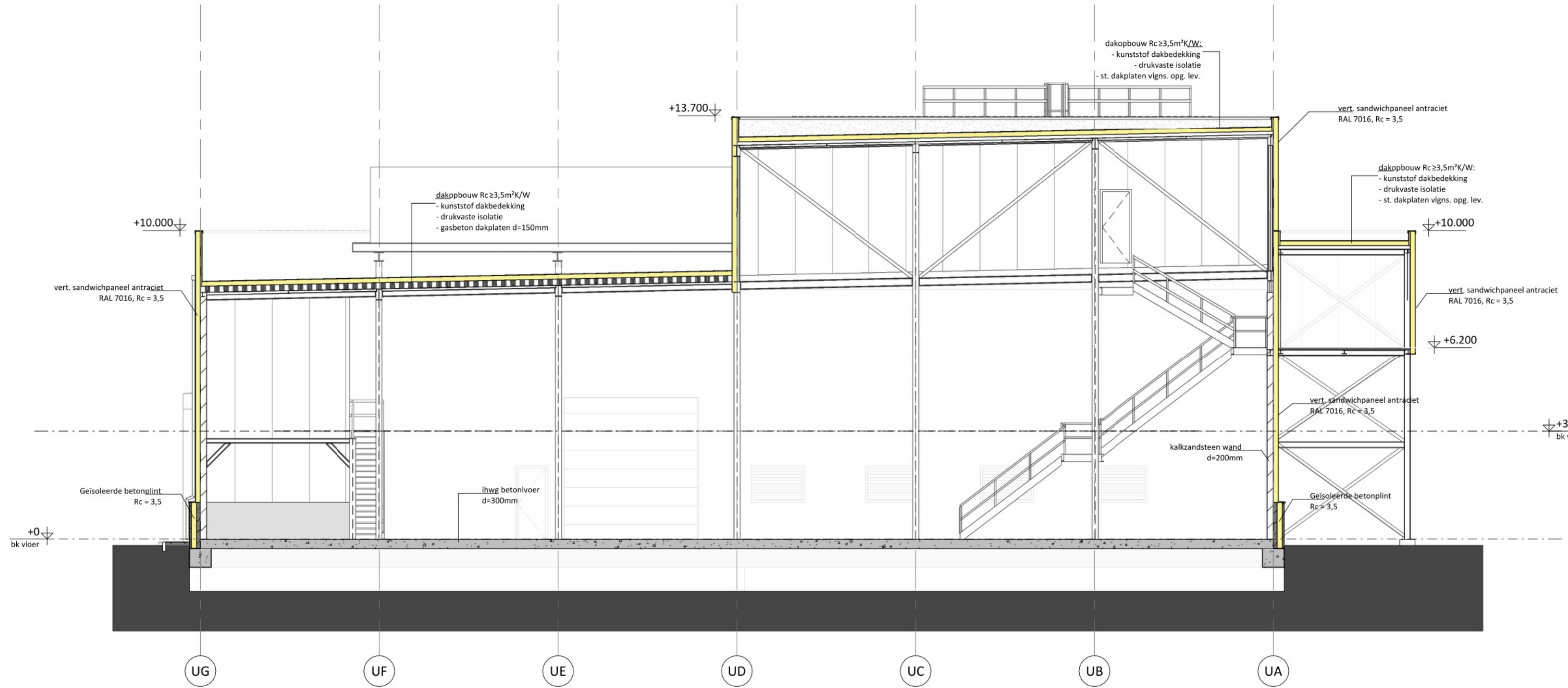
Doorsnede UB
