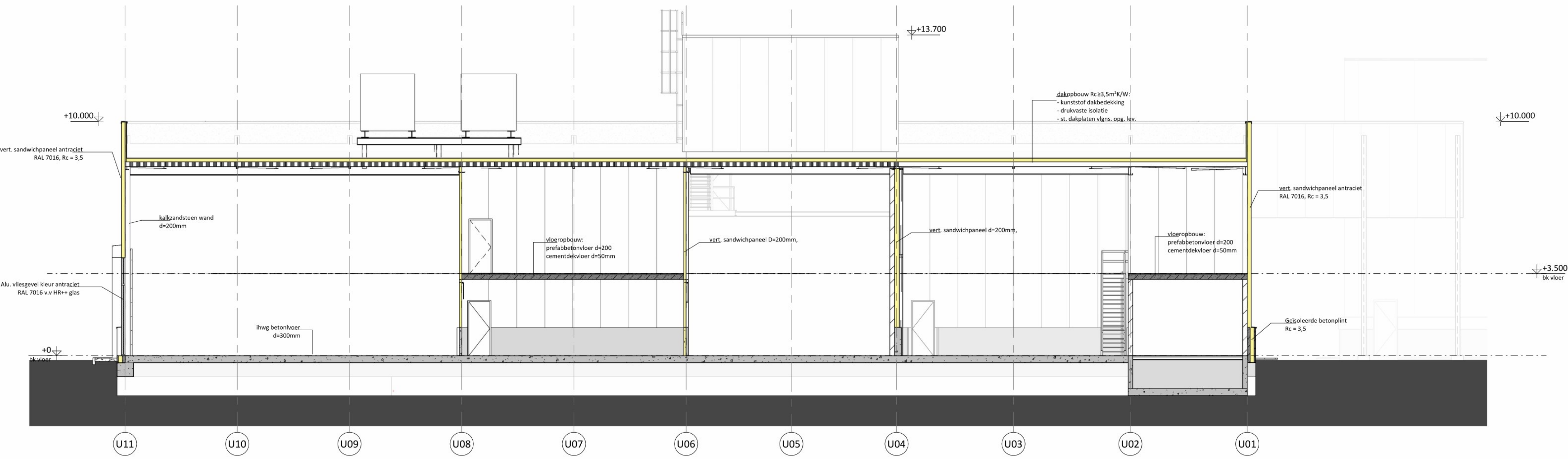
Doorsnede UA
