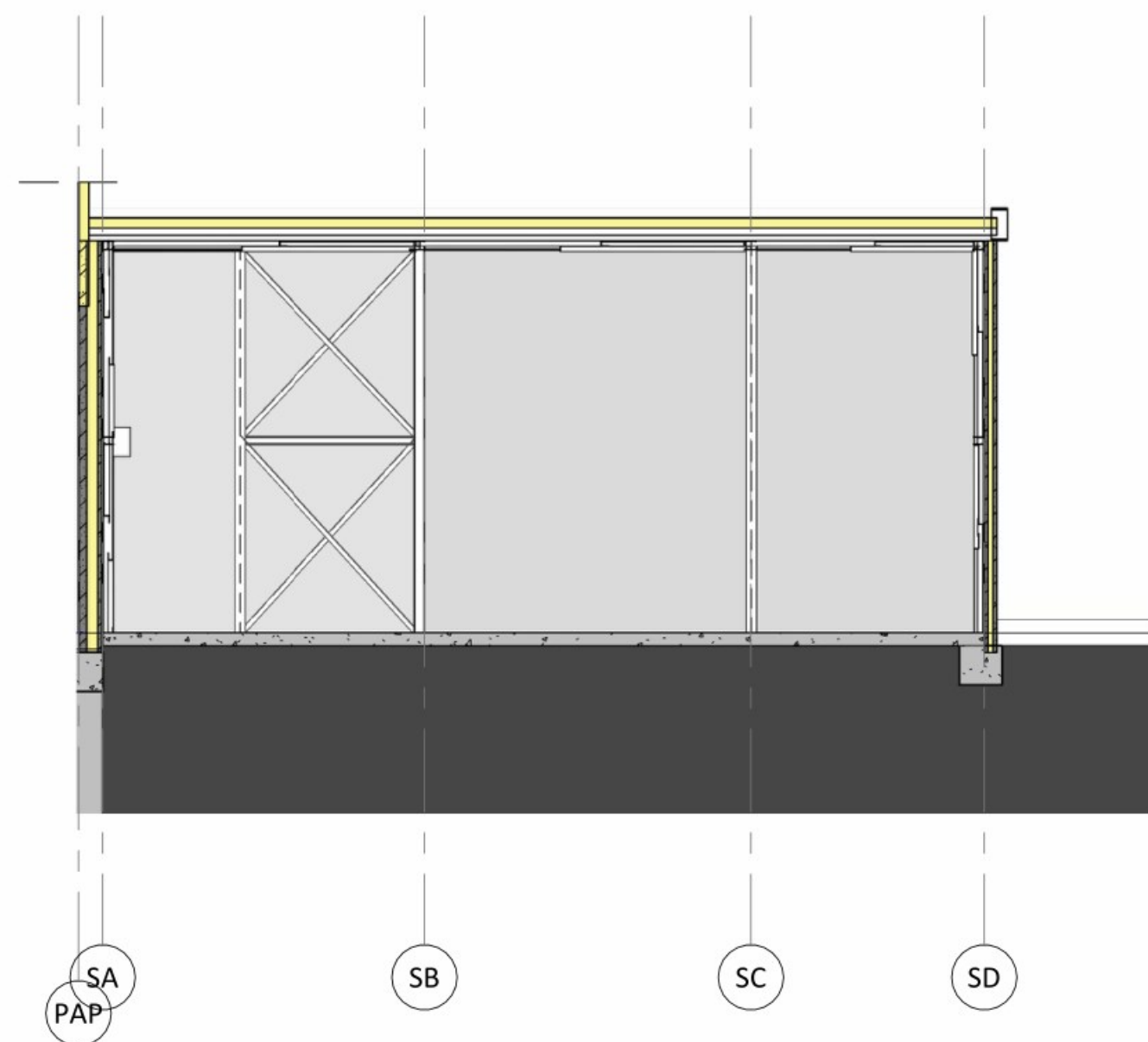
Doorsnde S1-A
