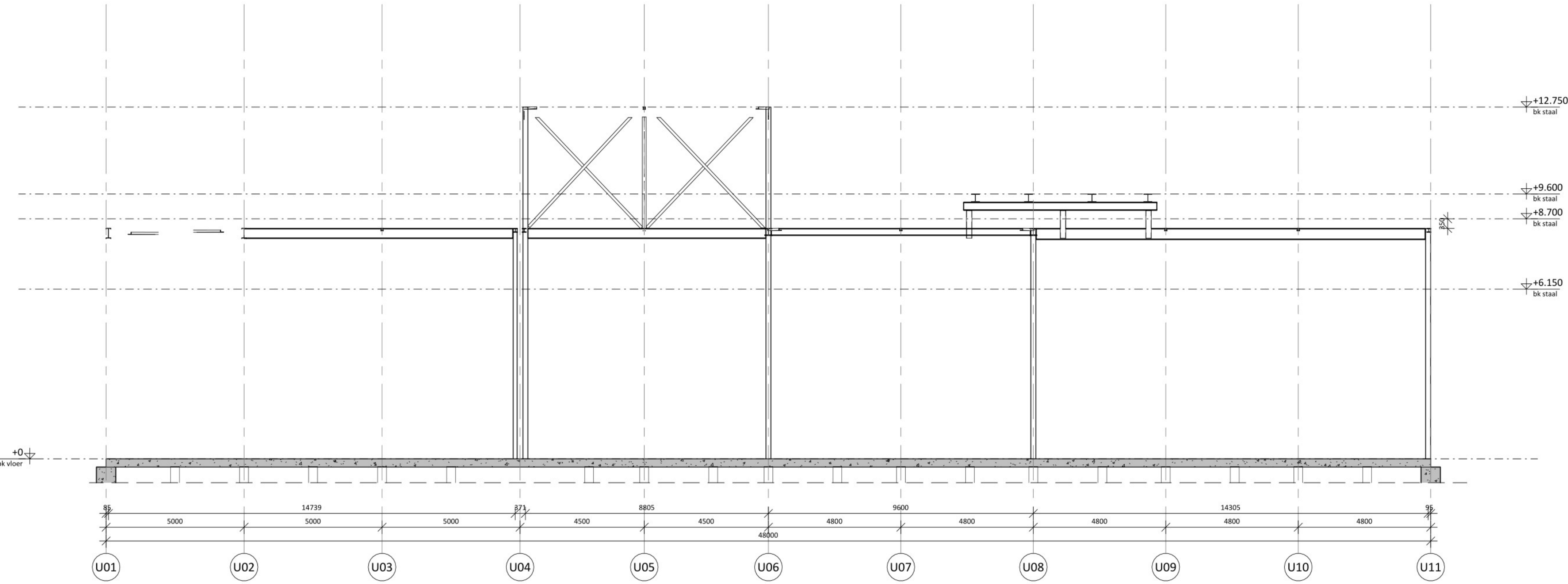
Doorsnede as UD Schaal: 1 : 100
