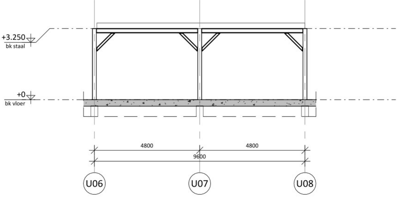
Doorsnede boven as UF Schaal: 1 : 100
