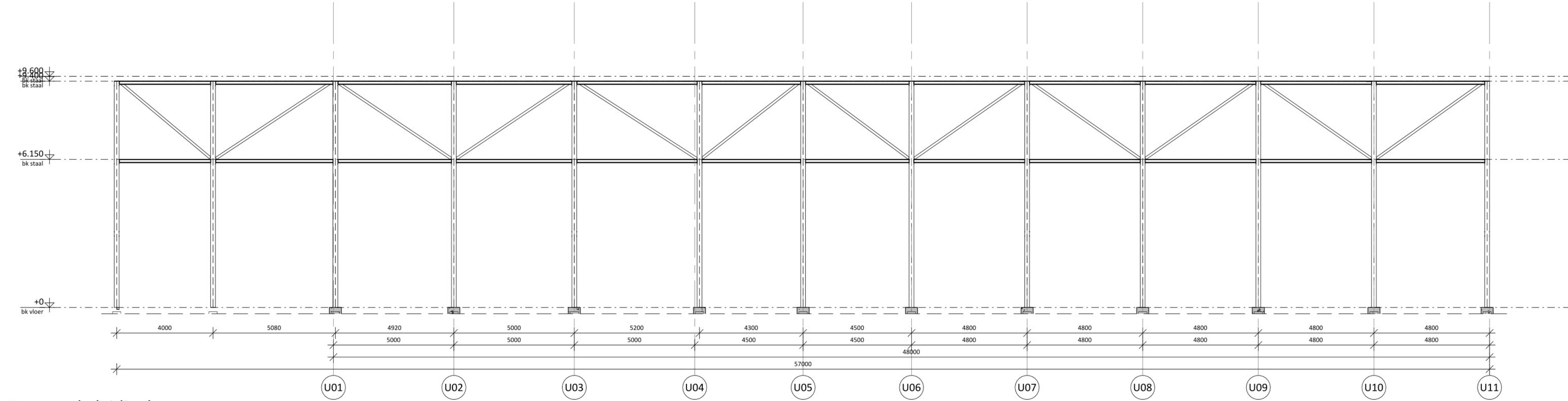
Doorsnede leidingbrug Schaal: 1 : 100
