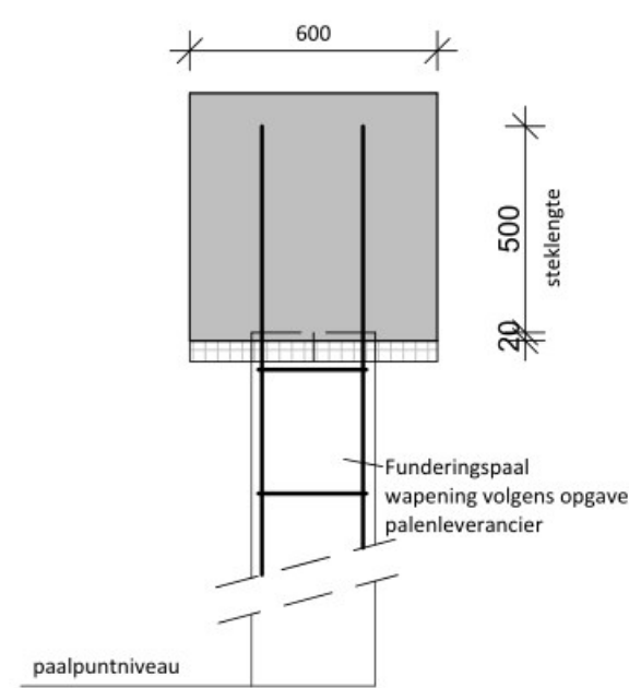
Principe detail funderingspaal Schaal: 1:20
