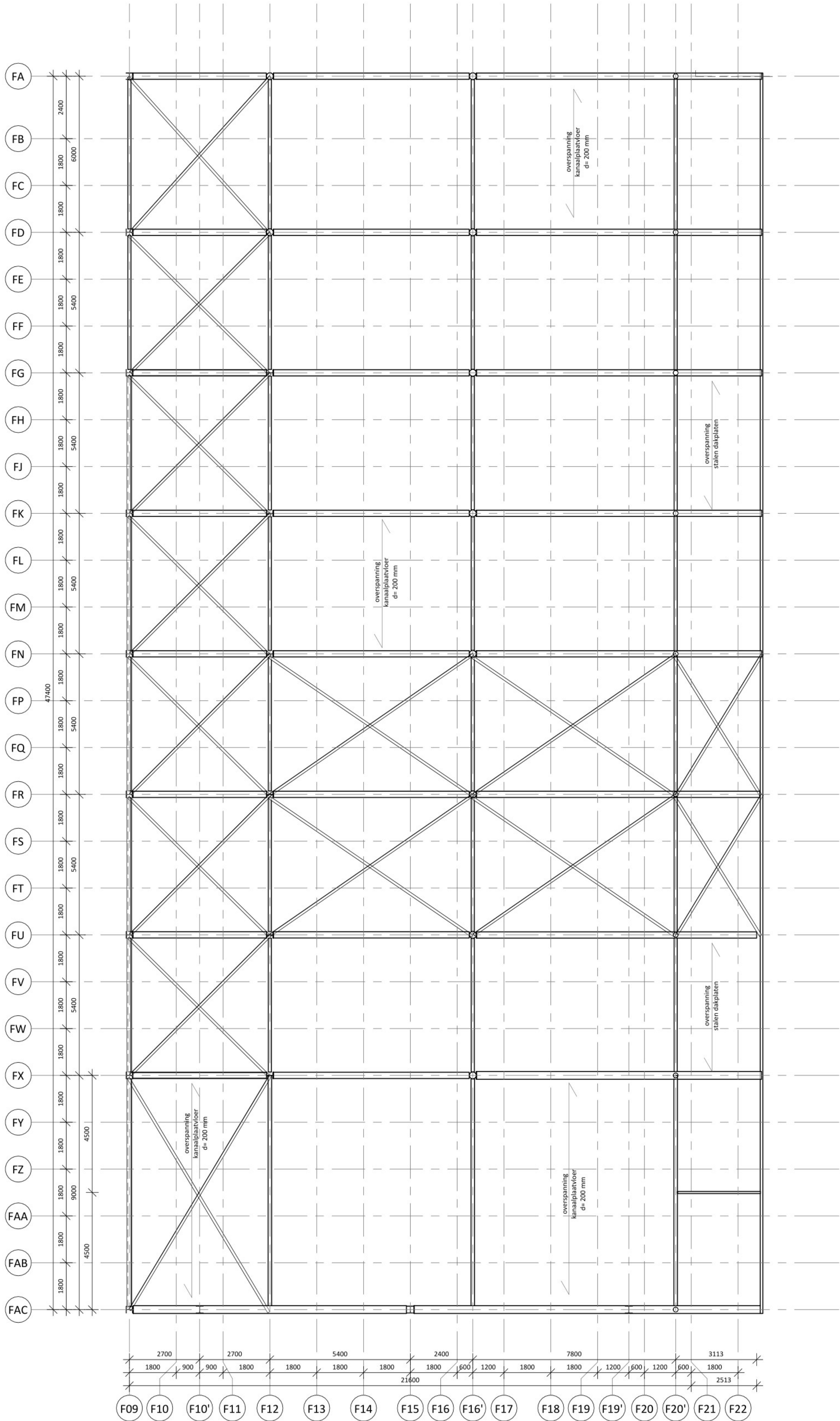
Staalconstructie hoge dak +5.000 Schaal: 1 : 100
