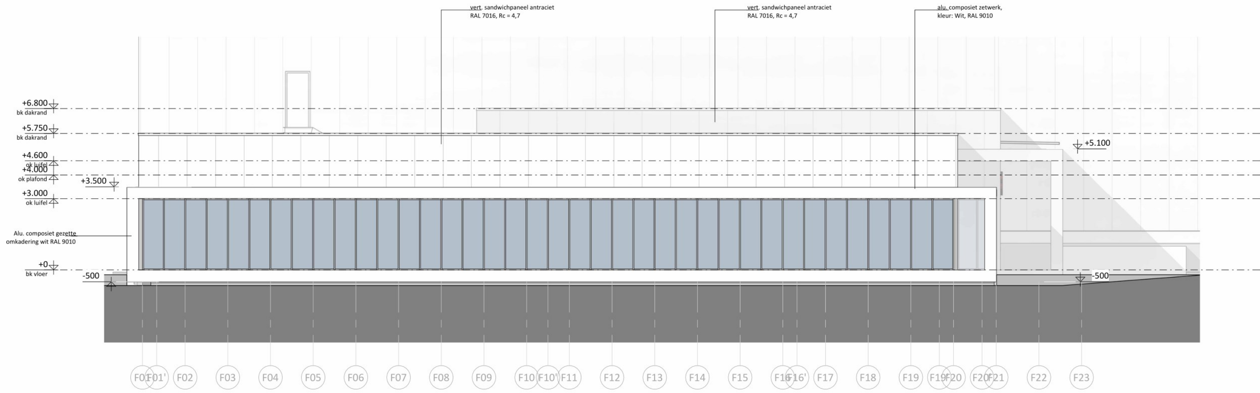
Zuidgevel faciliteiten
