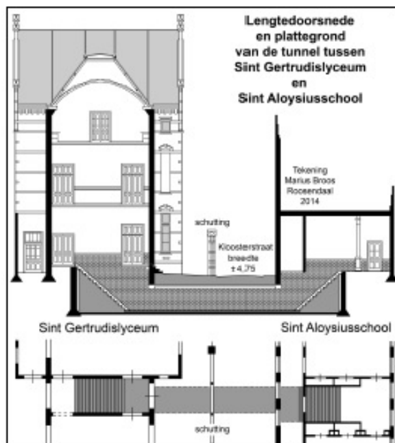
Lengtedoorsnede en plattegrond van de tunnel tussen het Sint Gertrudislyceum en de Sint Aloysiuschool. Tekening Marius Broos, Rosendaal.
