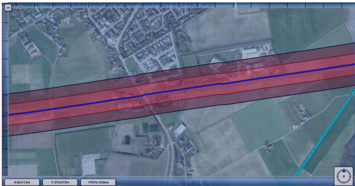
Figuur: Huidige ligging invloedsgebied (1% letaliteit) van de hogedruk aardgasleiding. De binnenste contour is de 100% letaliteitsafstand.
