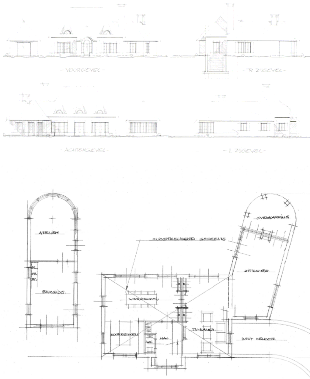
2.3: 3-d ontwerp en plattegrond nieuwe woning
