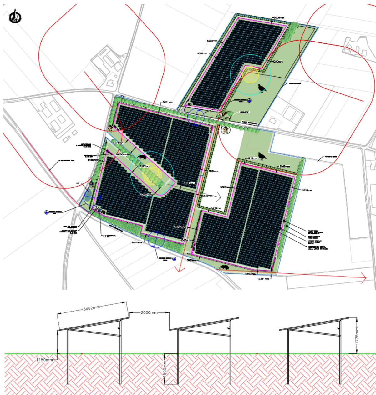
Afbeelding 1.Ontwerp en dwarsprofiel van de zonneweide.
