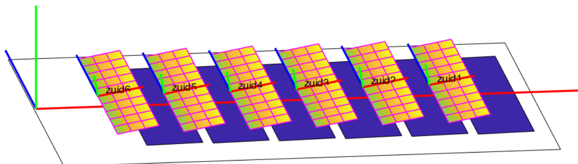
Afbeelding 6. Modelweergave van de gekozen eenzijdige zuid-zuid-west georiënteerde opstelling.
