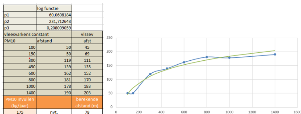
Figuur 5-5 berekening adviesafstand endotoxine
