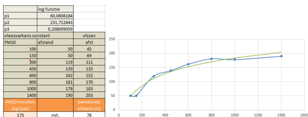
Figuur 5-8 Berekening adviesafstand endotoxine
