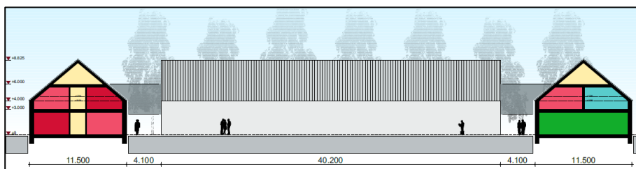
Afbeelding 3: Doorsnede
