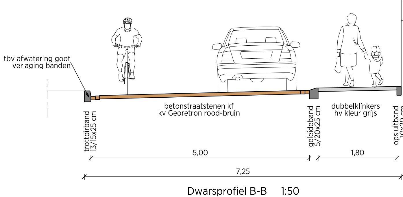
Dwarsprofiel B-B 1:50
