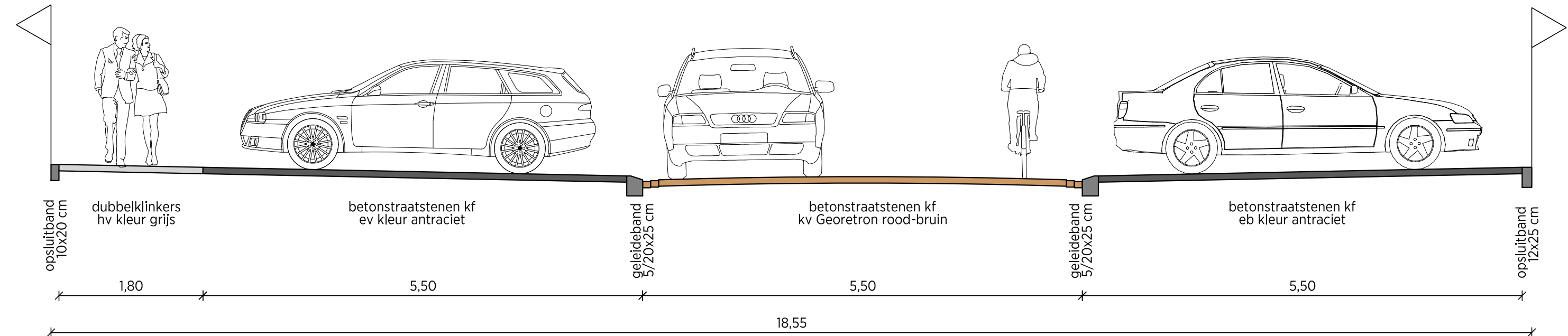
Dwarsprofiel A-A 1:50
