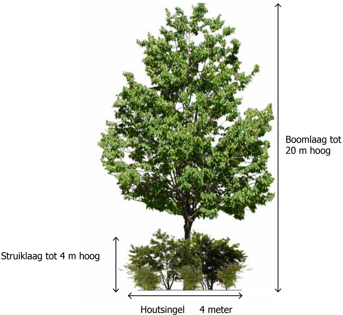
Doorsnede houtsingel
