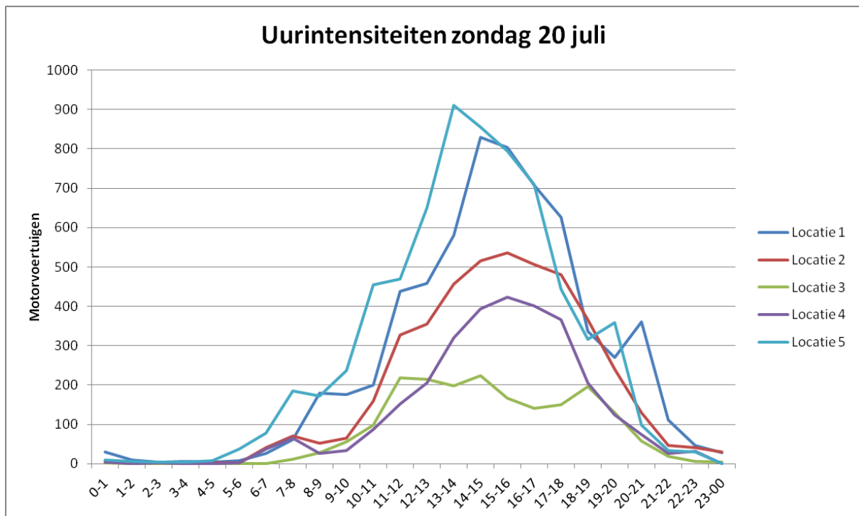
Figuur 2.5 Intensiteiten per uur zondag 20 juli 2014
