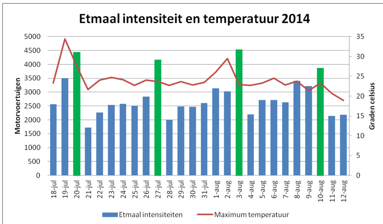
Figuur 4.3 intensiteiten en maximale temperaturen 2014
