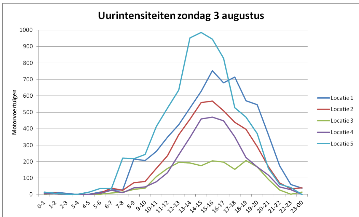
Figuur 2.6 Intensiteiten per uur zondag 3 augustus 2014
