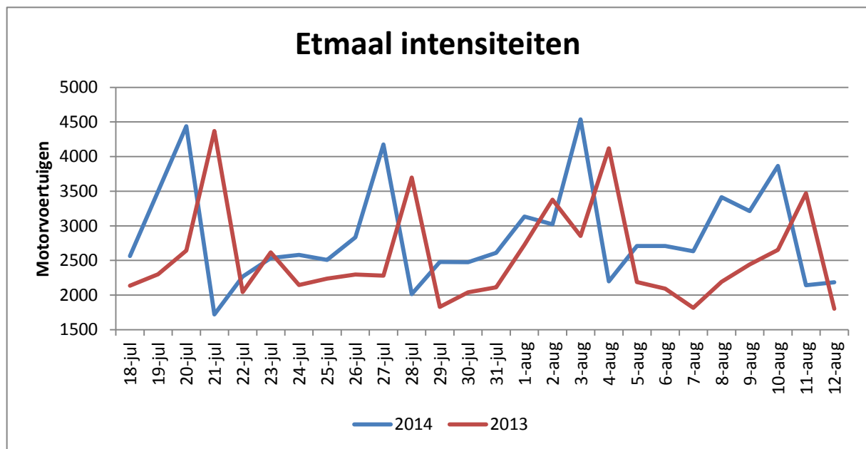
Figuur 4.1 Etmaal intensiteiten 2013, 2014
