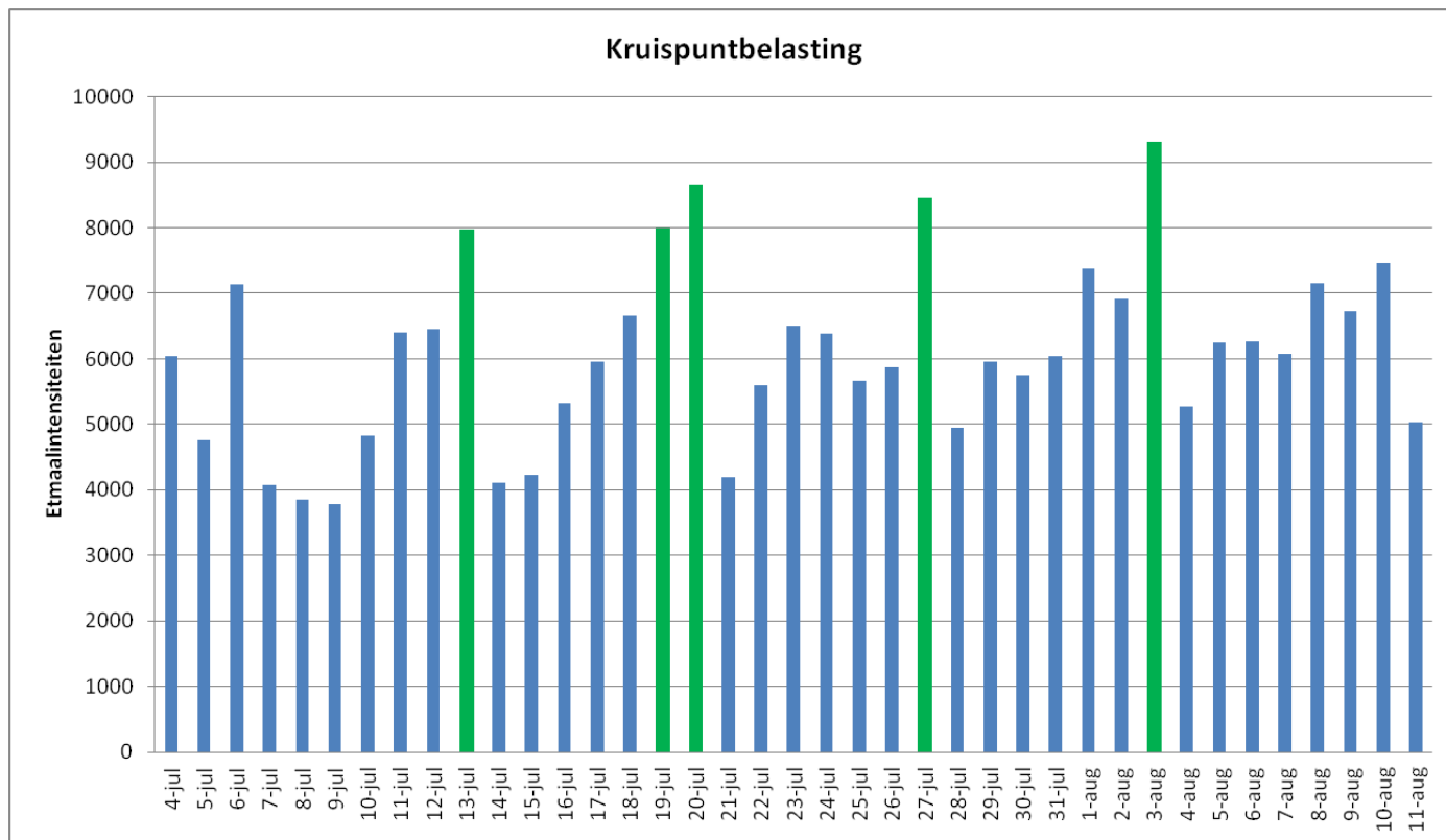
Figuur 2.4 Verkeersbelasting kruispunt N361 – Haven Lauwersoog tijdens onderzoeksperiode 2014
