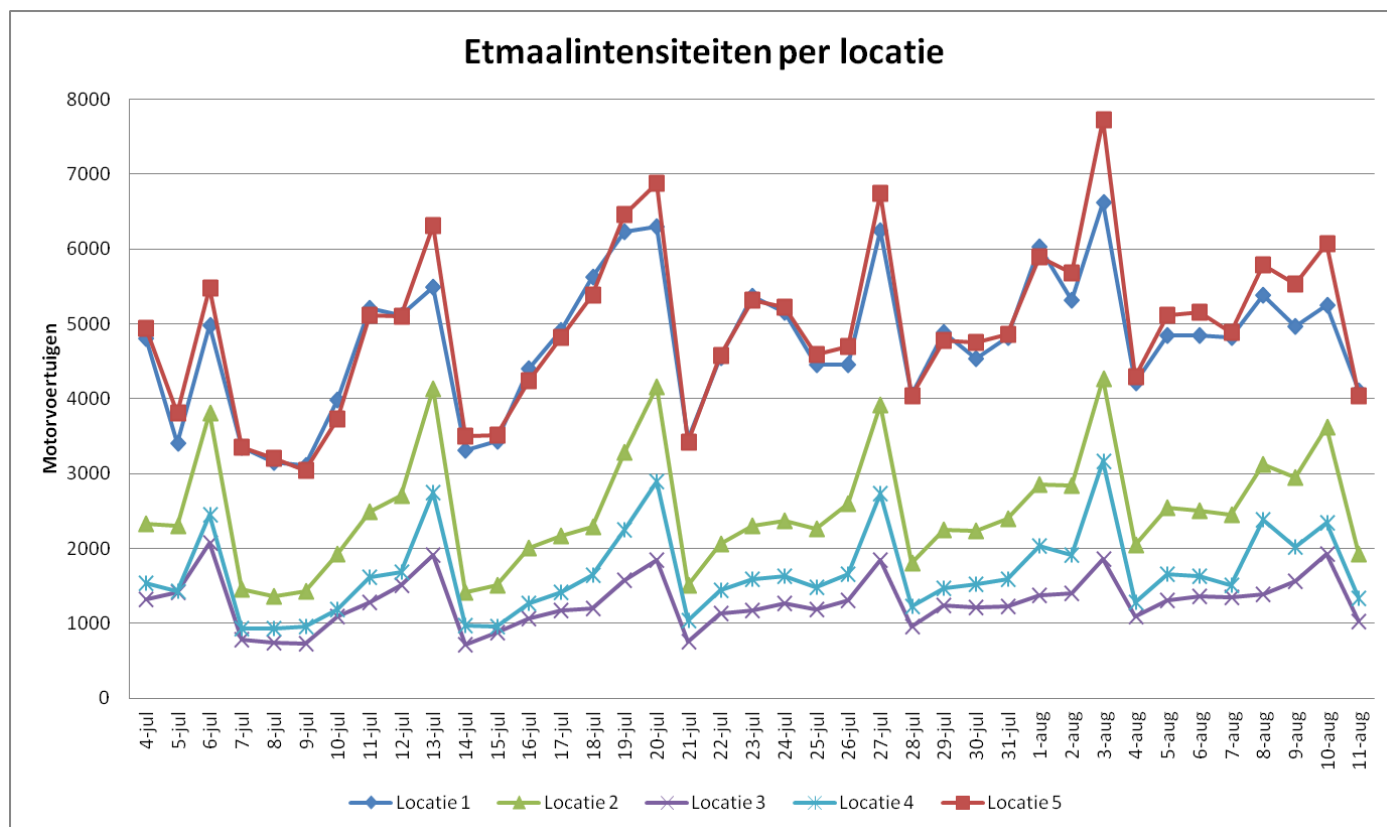
Figuur 2.3 Verloop etmaalintensiteiten onderzoeksperiode 2014
