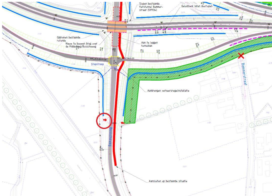
uitsnede van het Referentie Ontwerp (RO) N279 Veghel-Asten
