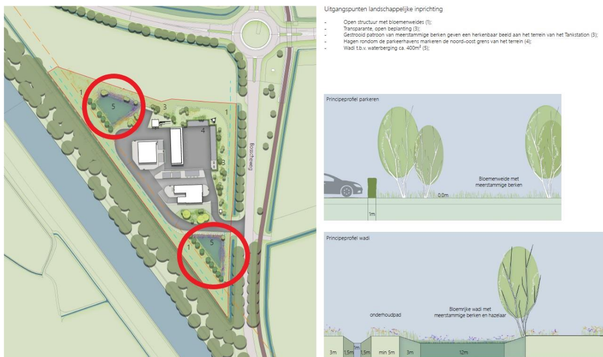
locatie WADI's (rood omcirkeld) op het terrein van het tankstation
