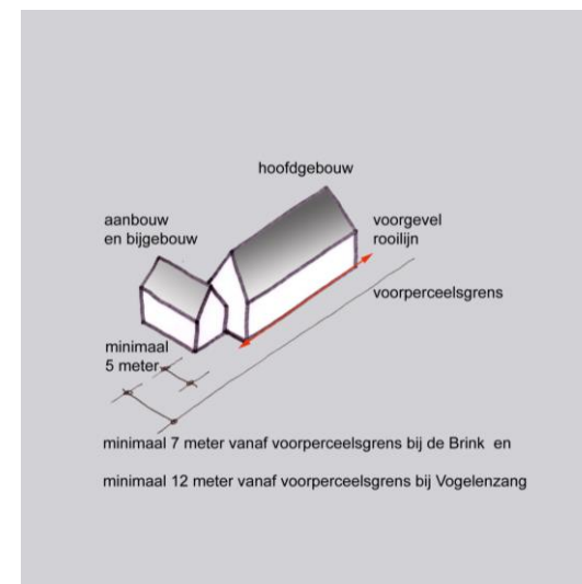
Situering bijgebouwen
