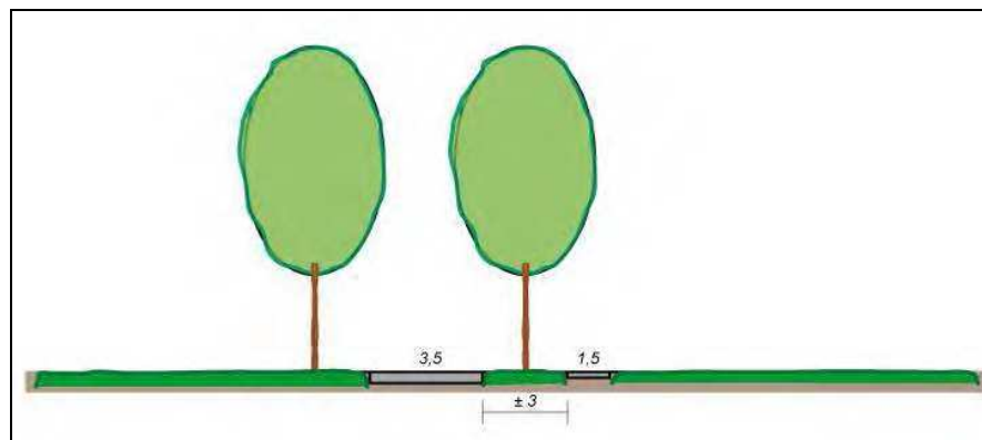
Profiel hoofdwegenstructuur
