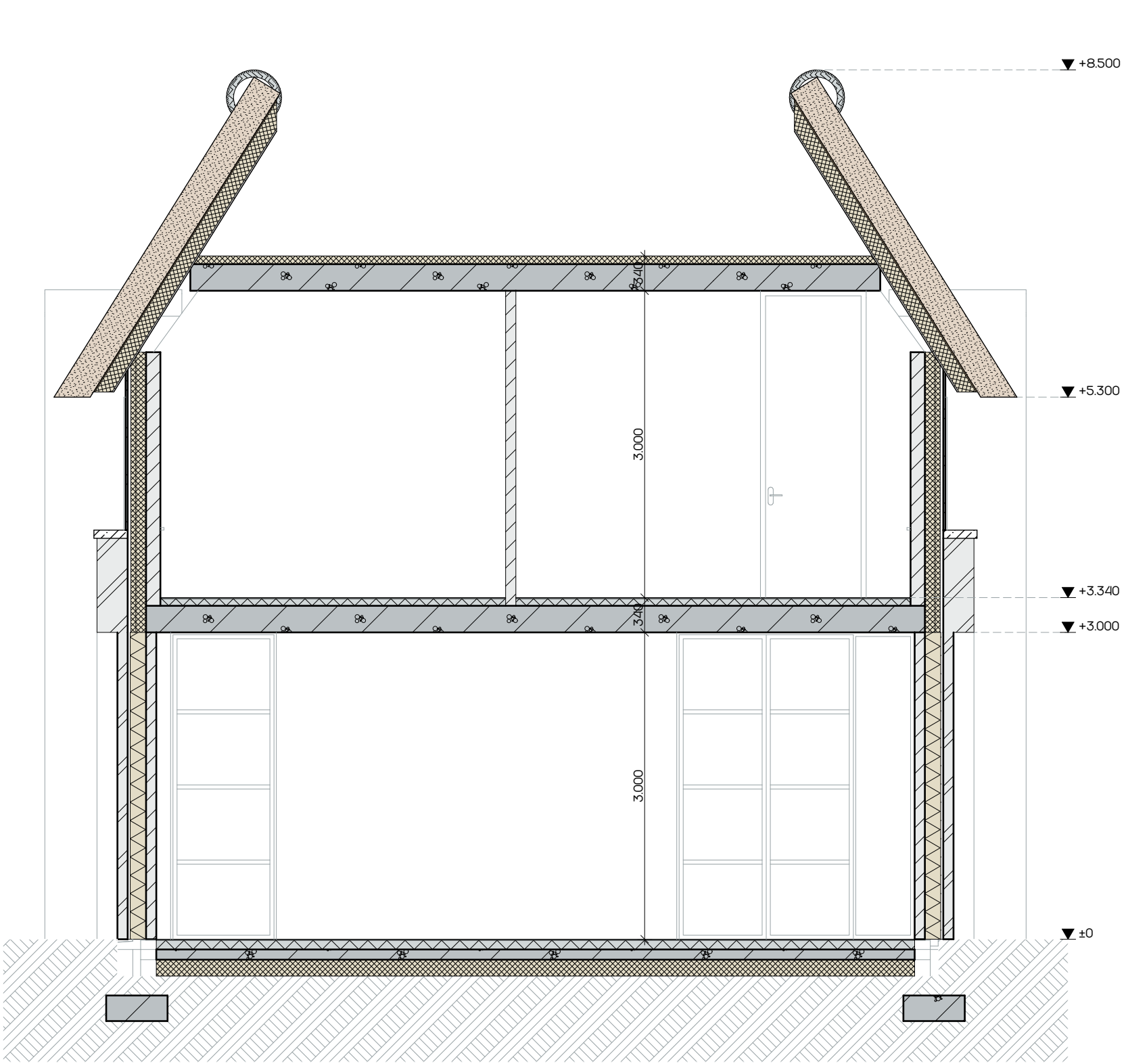
Doorsnede B-B
