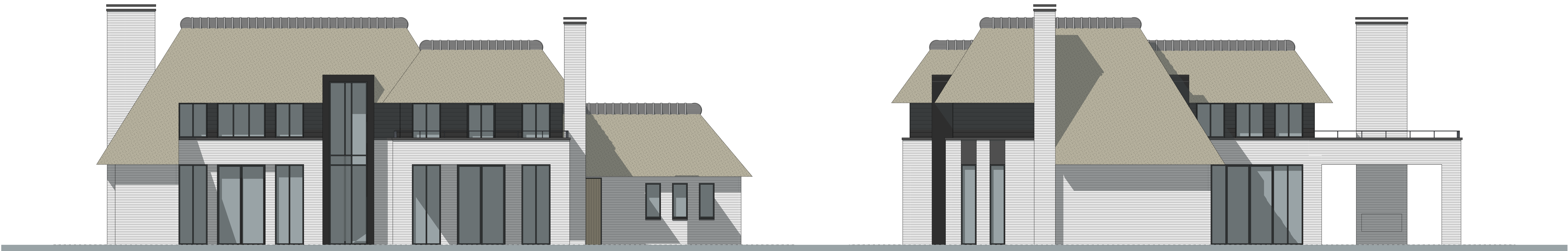
ACHTERGEVEL
