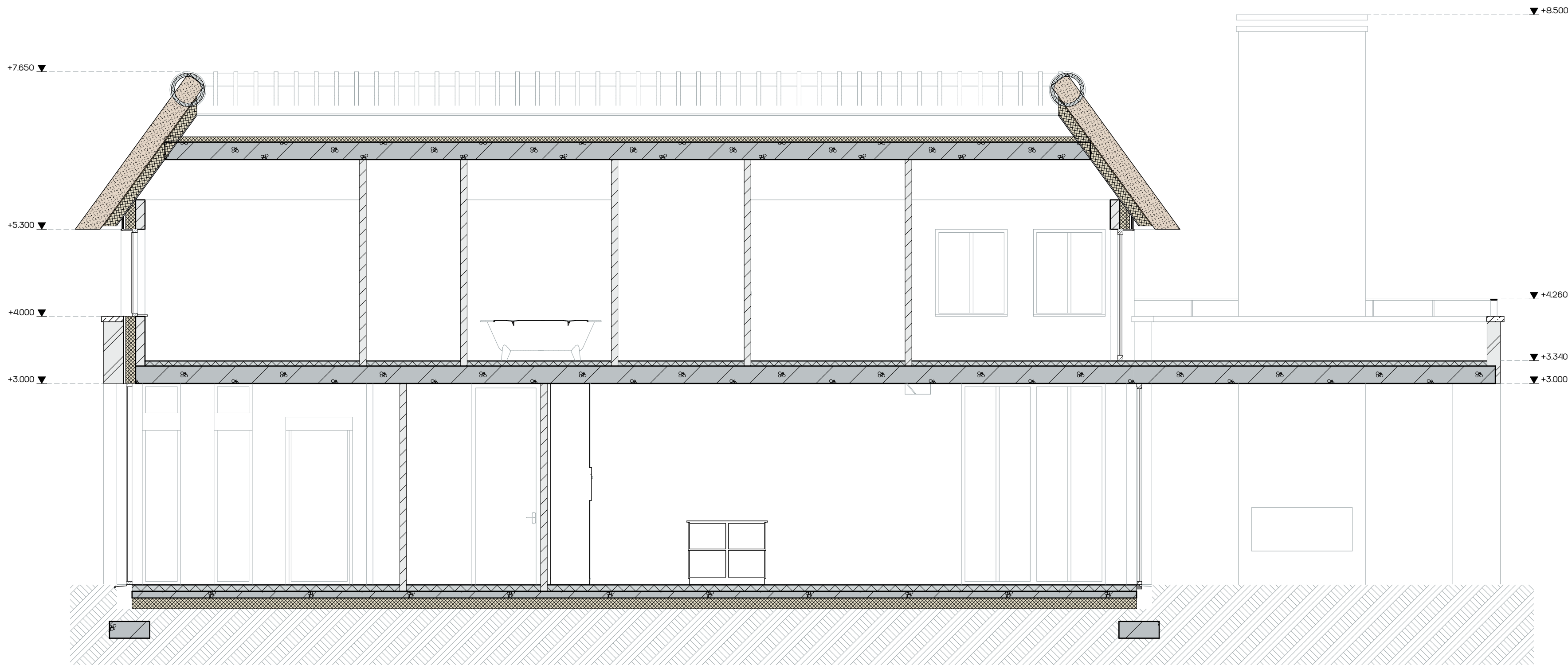
Doorsnede C-C
