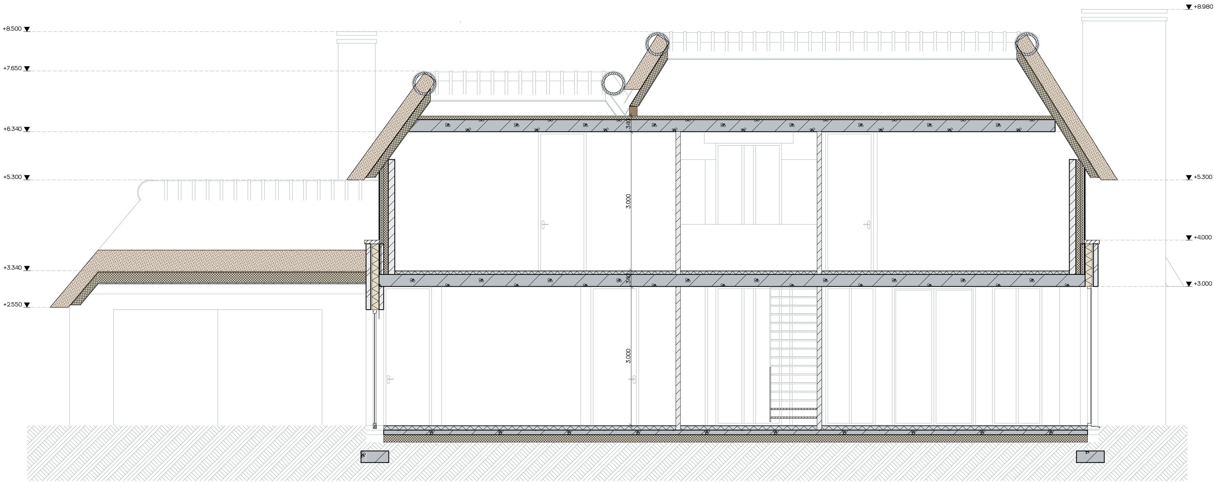
Doorsnede A-A
