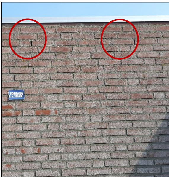
Figuur 16. Twee open stootvoegen in de gevel van het zorgcentrum, aangegeven met een rode cirkel.
