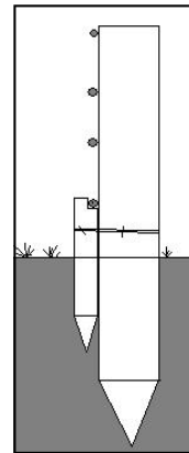
Zijaanzicht ankerpaal.
