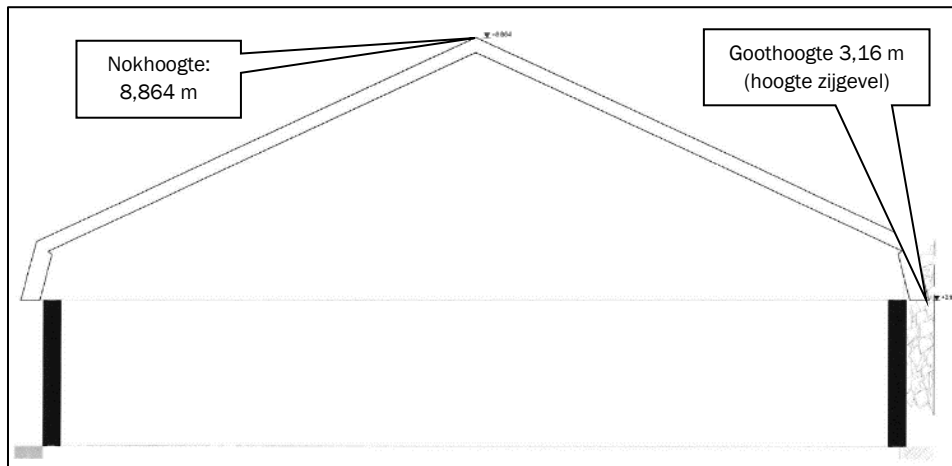
Figuur 10: Impressie dak-gevelverhouding nieuwe loods
