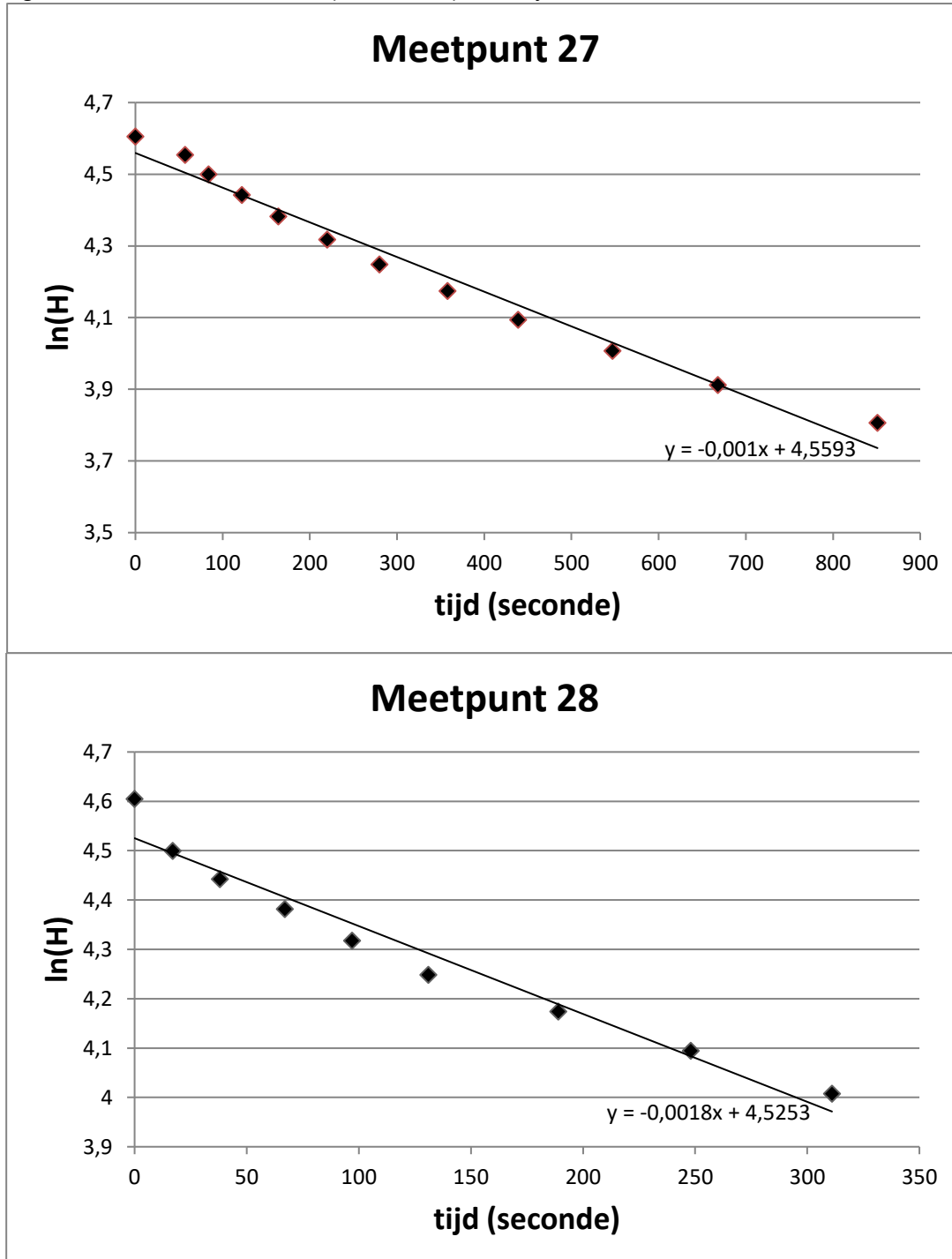
Figuur 4: Lineaire relatie tussen \ln(\text{waterkolom}) en de tijd
