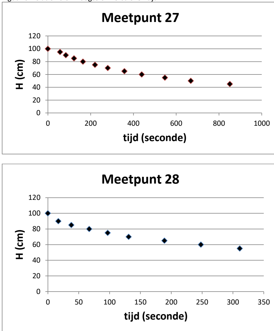
Figuur 3: relatie kolomhoogte en verstreken tijd
