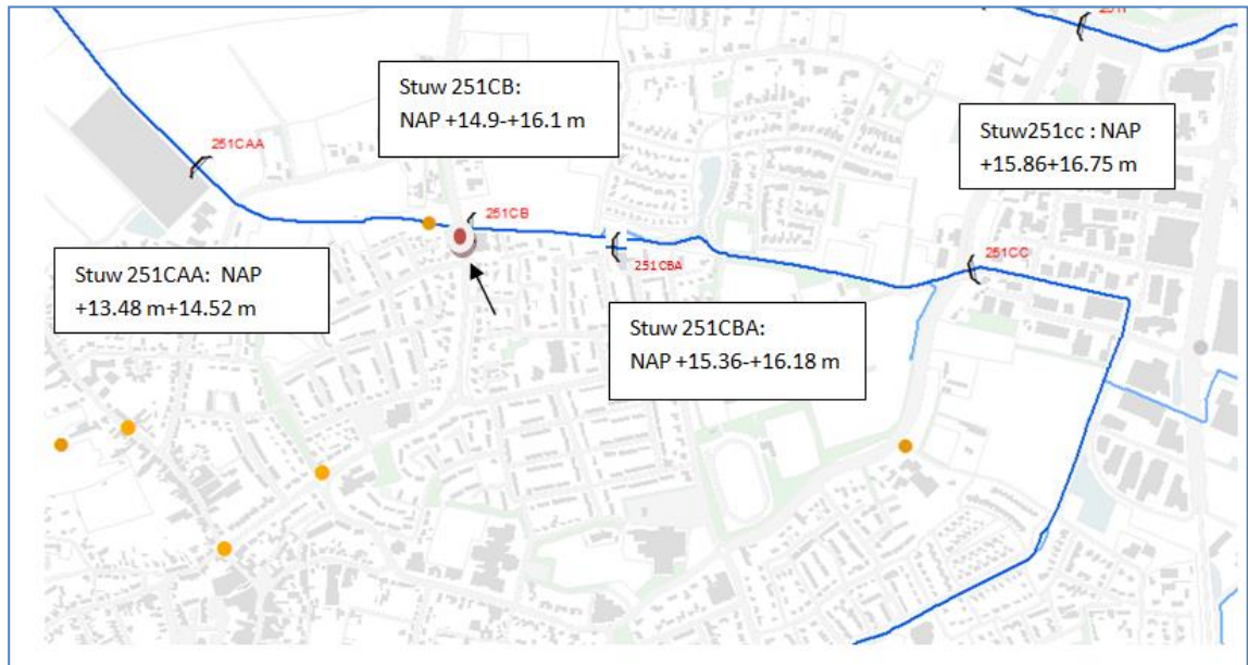
Figuur 1: gegevens stuwen Molenbroekseloep
