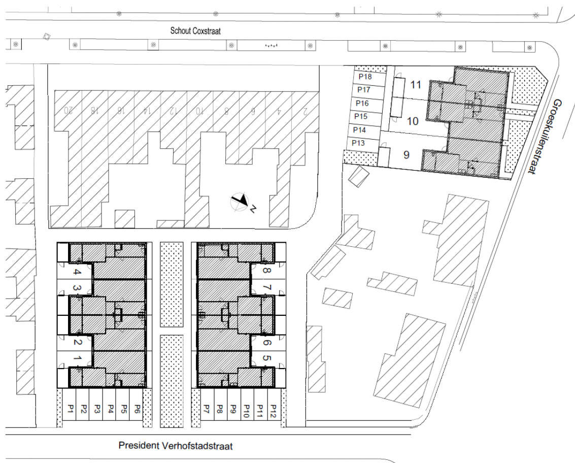
Figuur 2: Situatietekening
