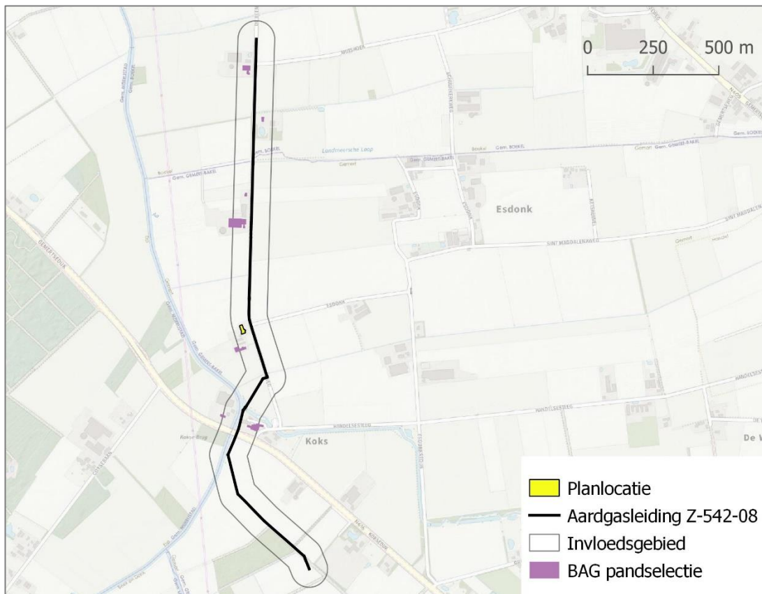
Figuur 5. BAG-pandselectie
