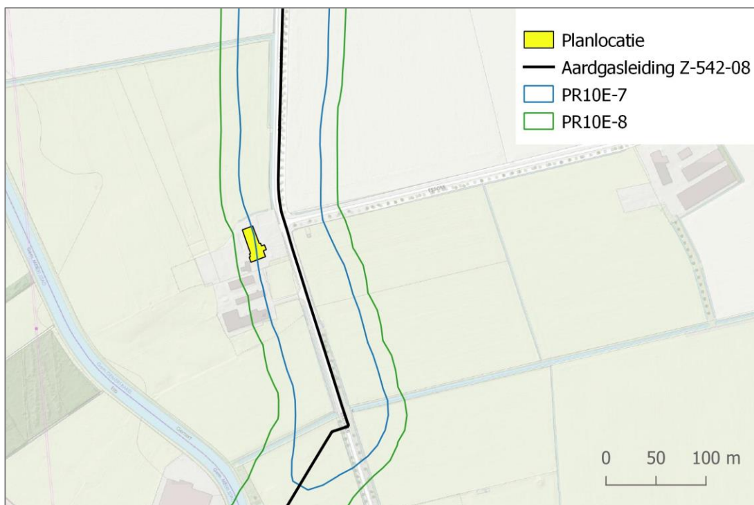
Figuur 3. PR-contouren aardgasleiding Z-542-08
