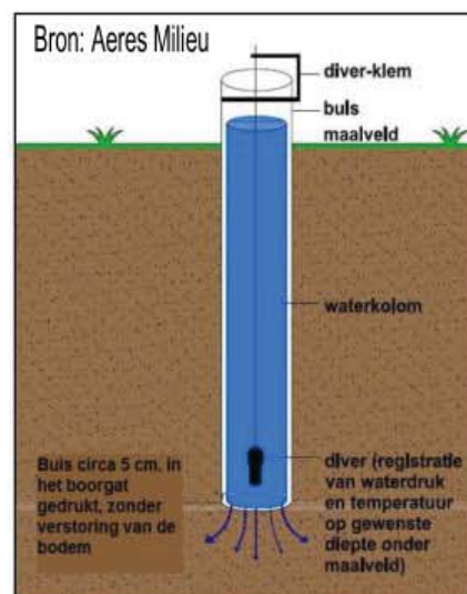
Afbeelding 5: Principetekening Open-end-test
