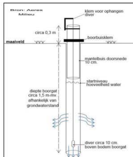
Afbeelding 6: Principetekening Porchettest
