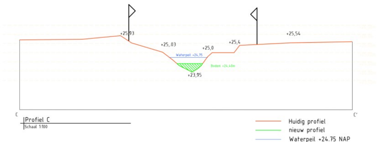
Figuur 18: Huidig en nieuw profiel van de Snelleloop bovenstrooms
