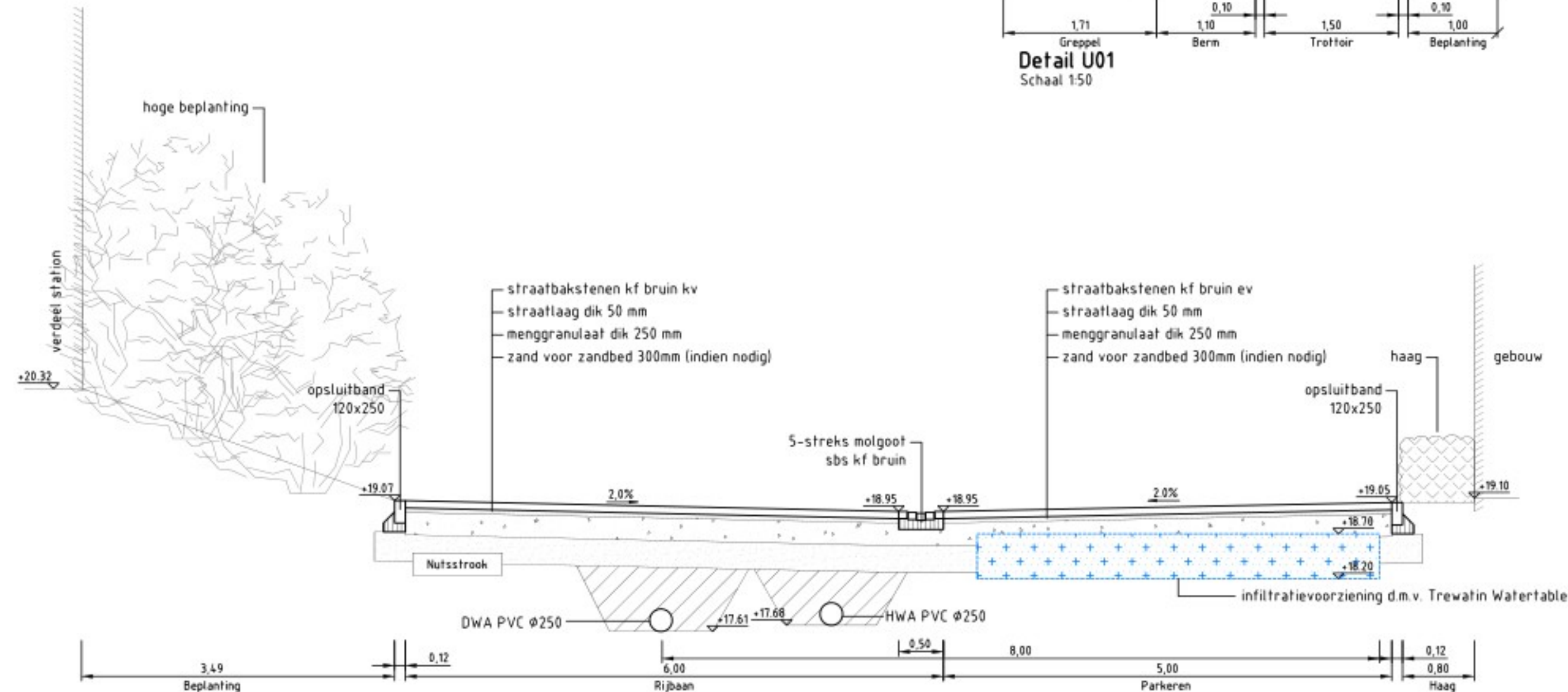
Dwarsprofiel C-C Schaal 1:50
