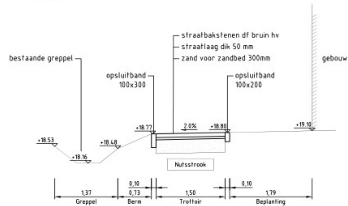
Dwarsprofiel B-B Schaal 1:50
