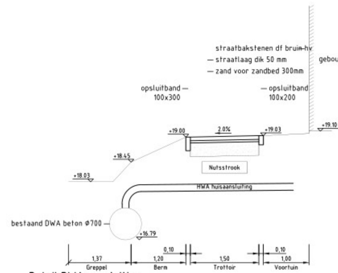
Detail DWA aansluiting Schaal 1:50
