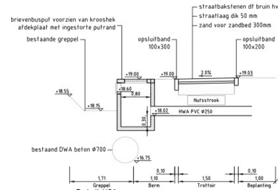
Detail U01 Schaal 1:50
