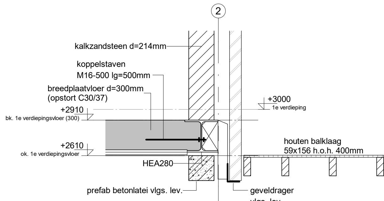
- D1.02 - (schaal 1 : 20)
