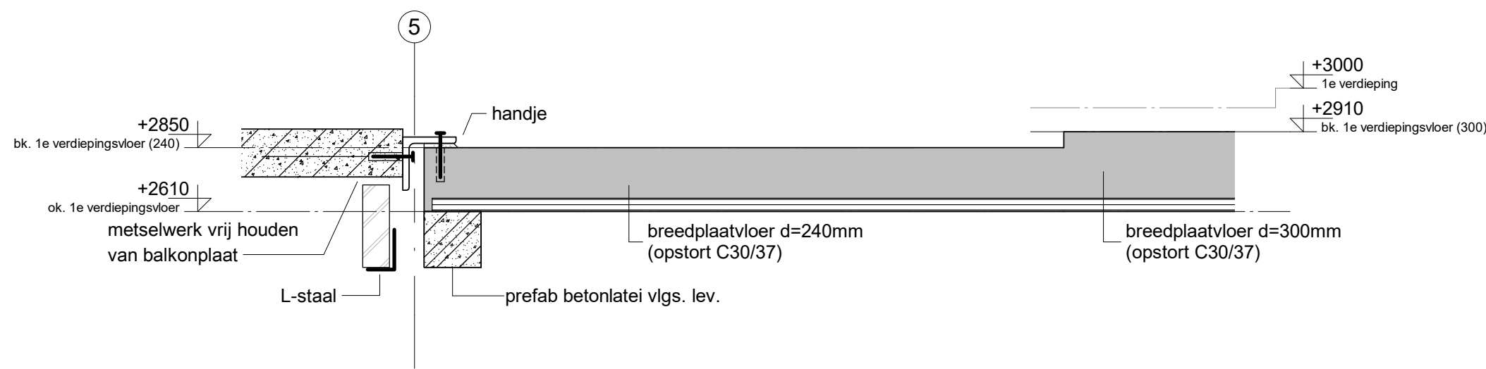
- D1.01 - (schaal 1 : 20)
