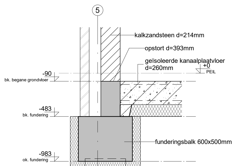
- D0.01 - (schaal 1 : 20)
