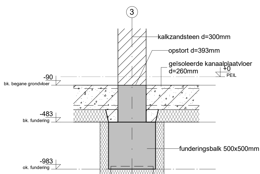
- D0.02 - (schaal 1 : 20)
