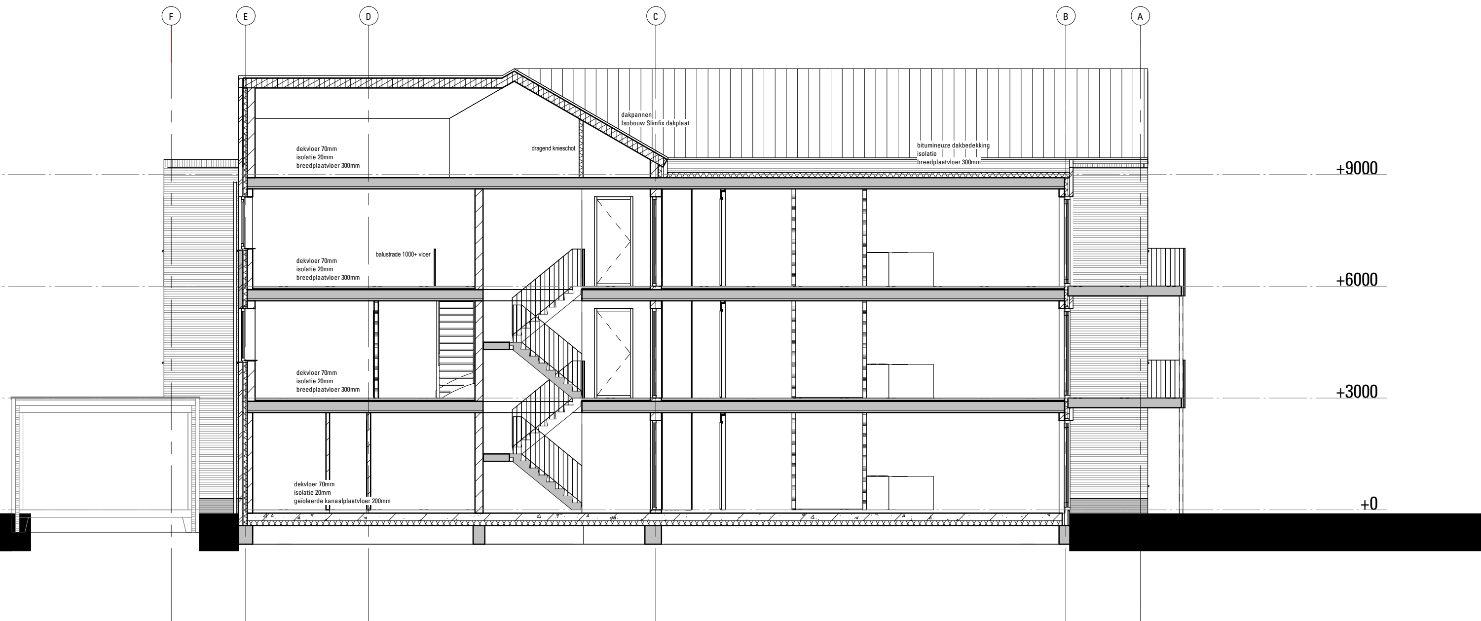
Doorsnede B
