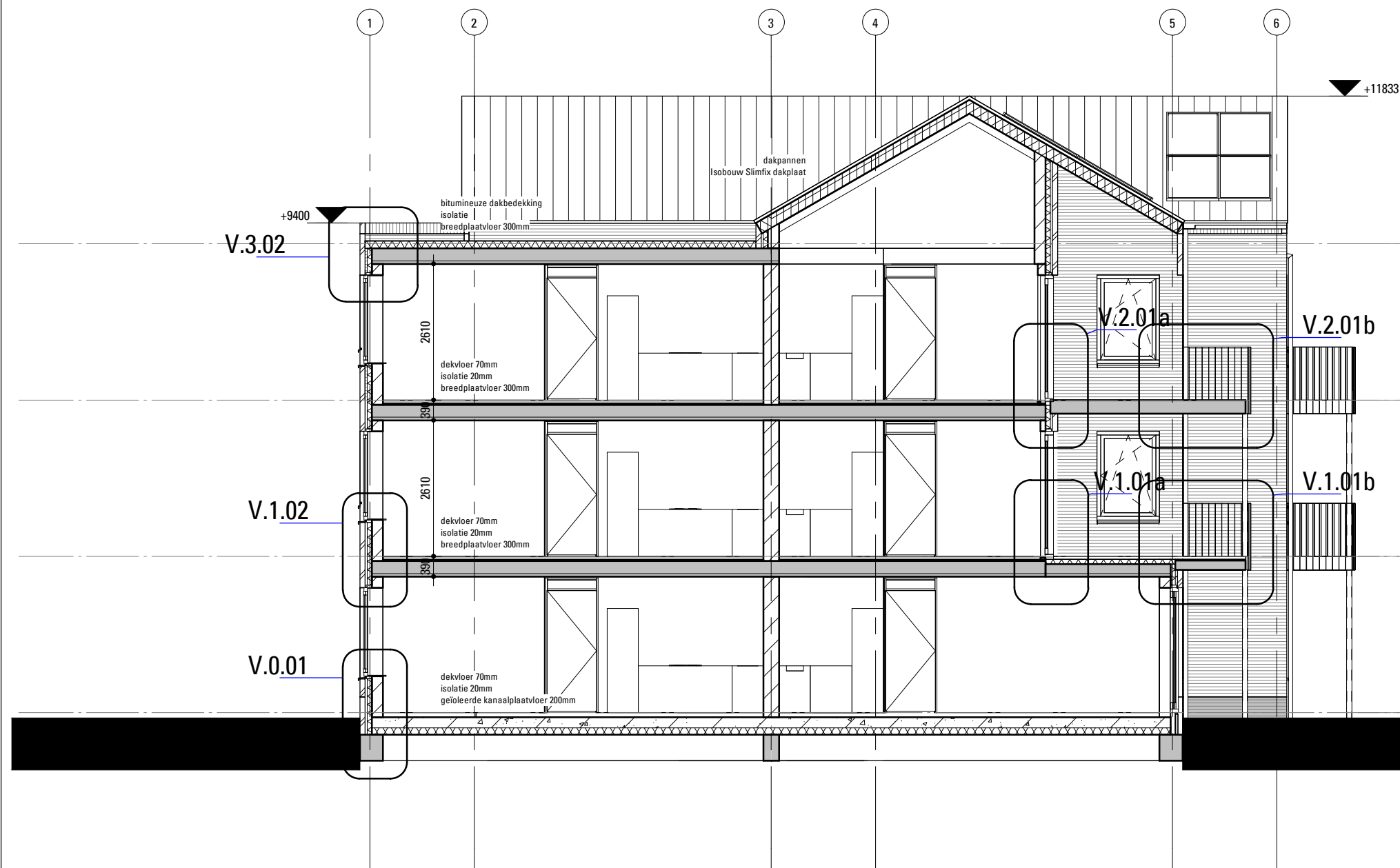
Doorsnede A
