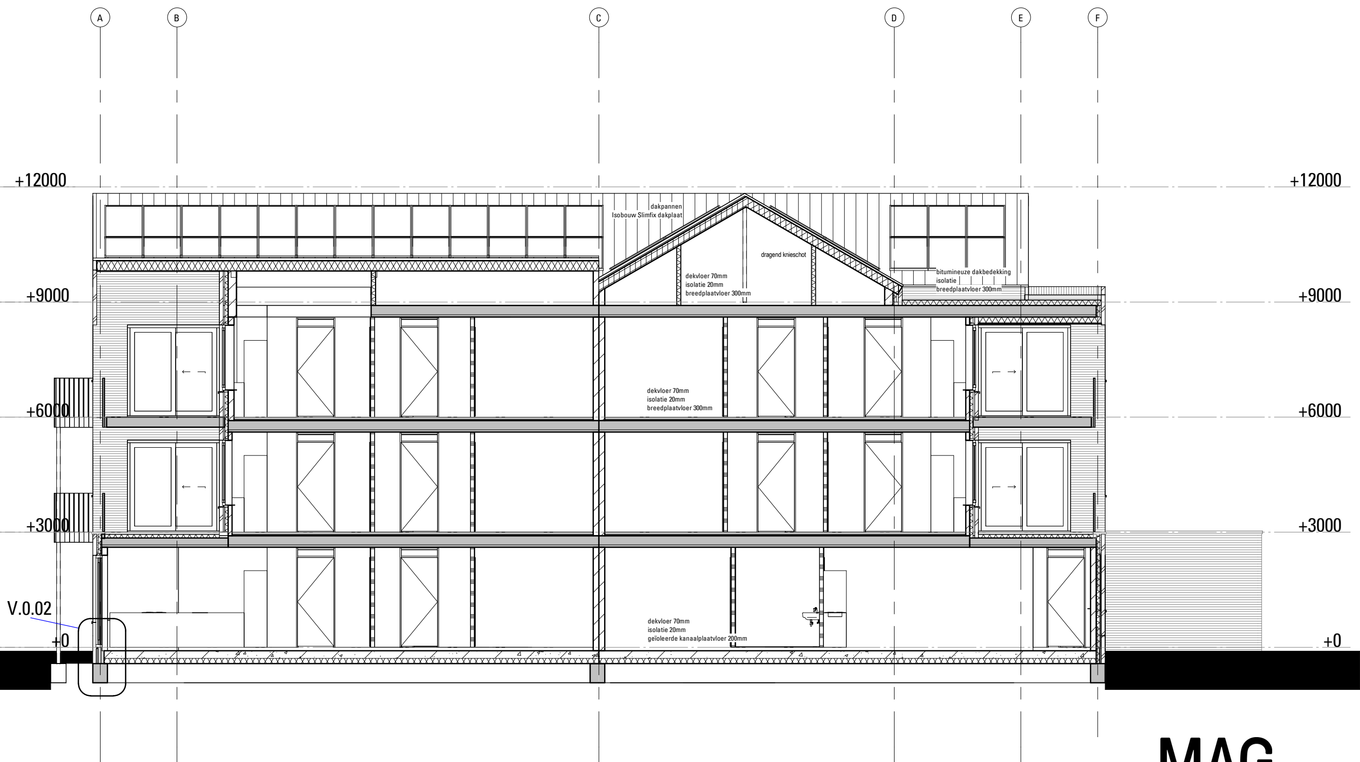
Doorsnede D
