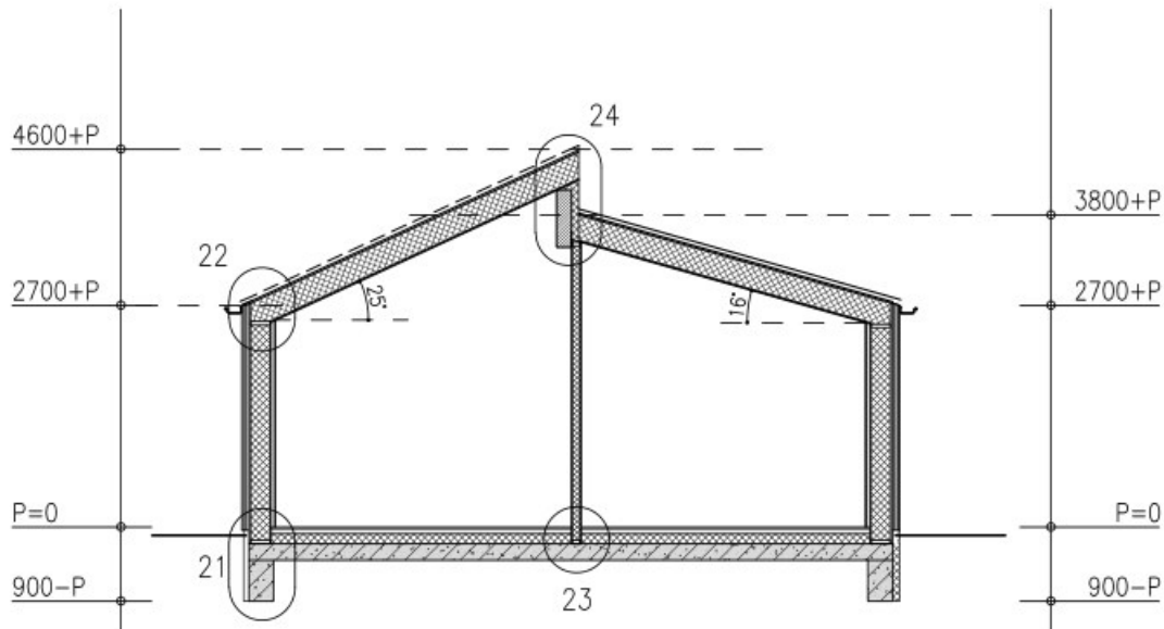
doorsnede A-A
