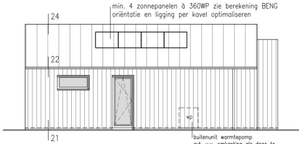
zijgevel links
