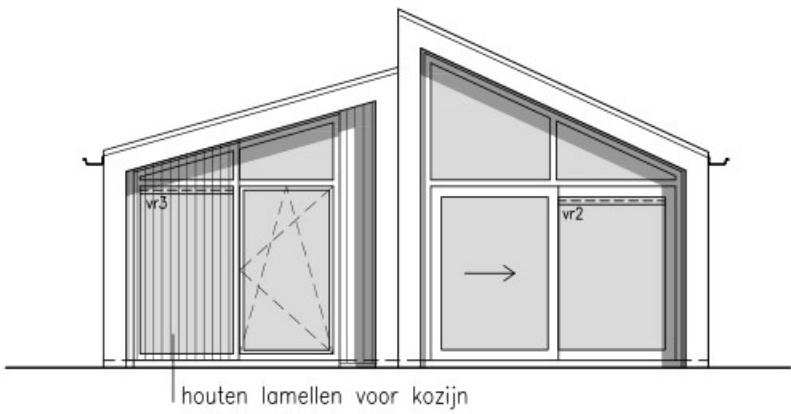
achtergevel
